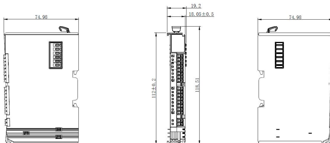
图 4.1 ZDM-C0800I 产品尺寸
