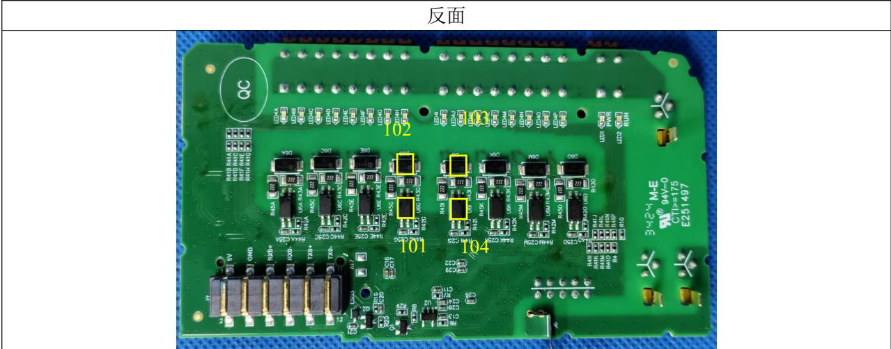
图 6 试验端口与试验点（黄色方框所示）
