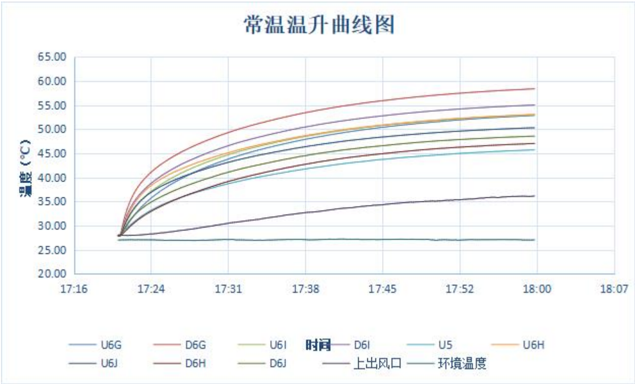
图 7 常温温升曲线图
