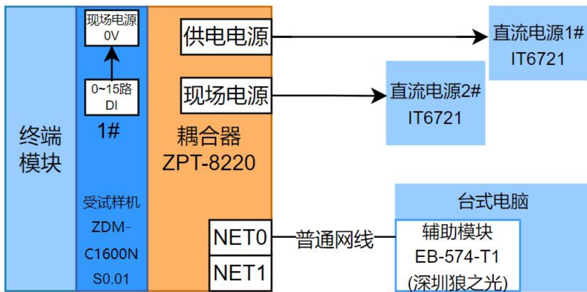
图 4 试验配置框图
