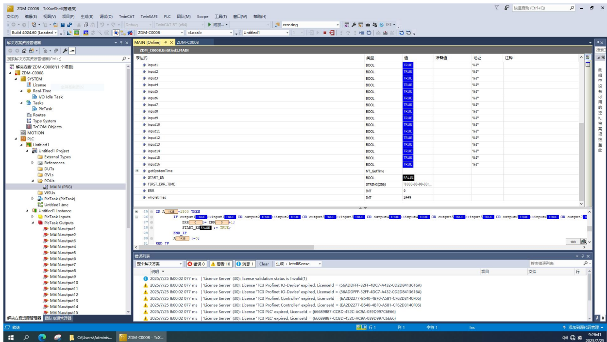
图 12 样机在湿热试验时第一次启动运行检查功能正常（24VDC 供电）
