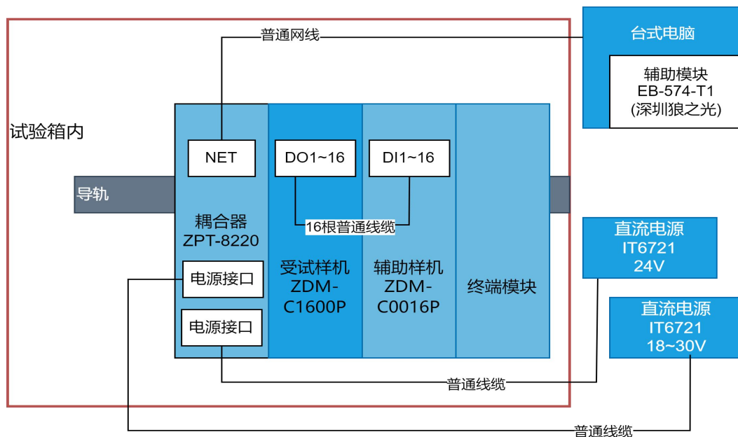
图 2 试验配置框图
