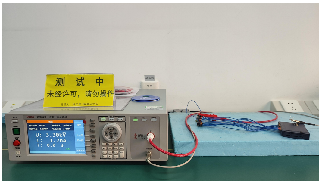
图 8 抗电强度试验 (DC)
