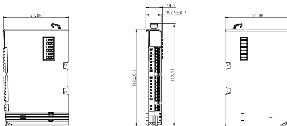
图 4.1 ZDM-C1600P 产品尺寸
