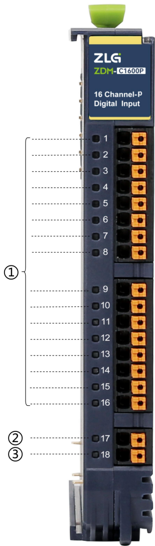
图 2.2 指示灯面板
