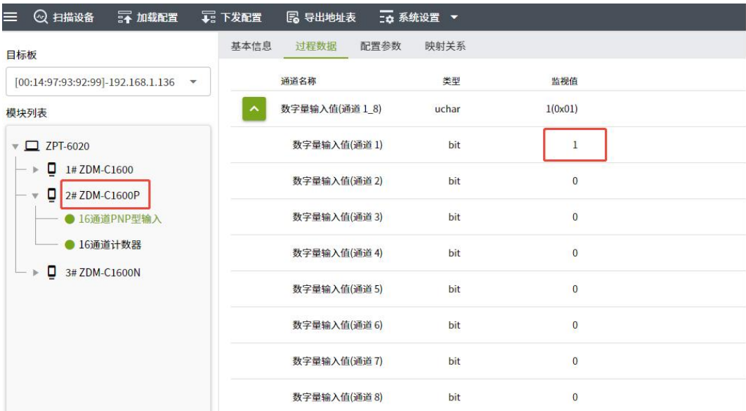
图 6.2 查看输入状态
