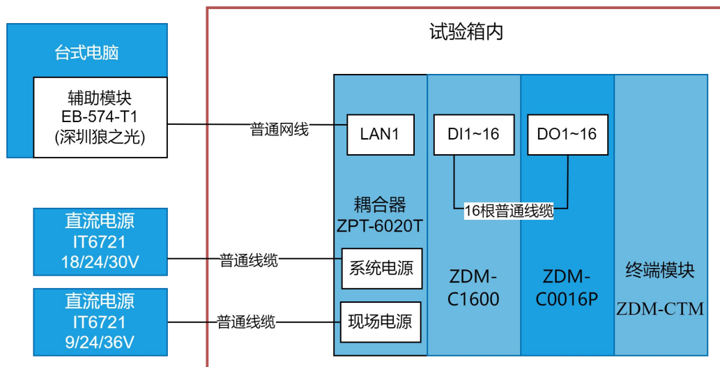
图 2 试验配置框图
