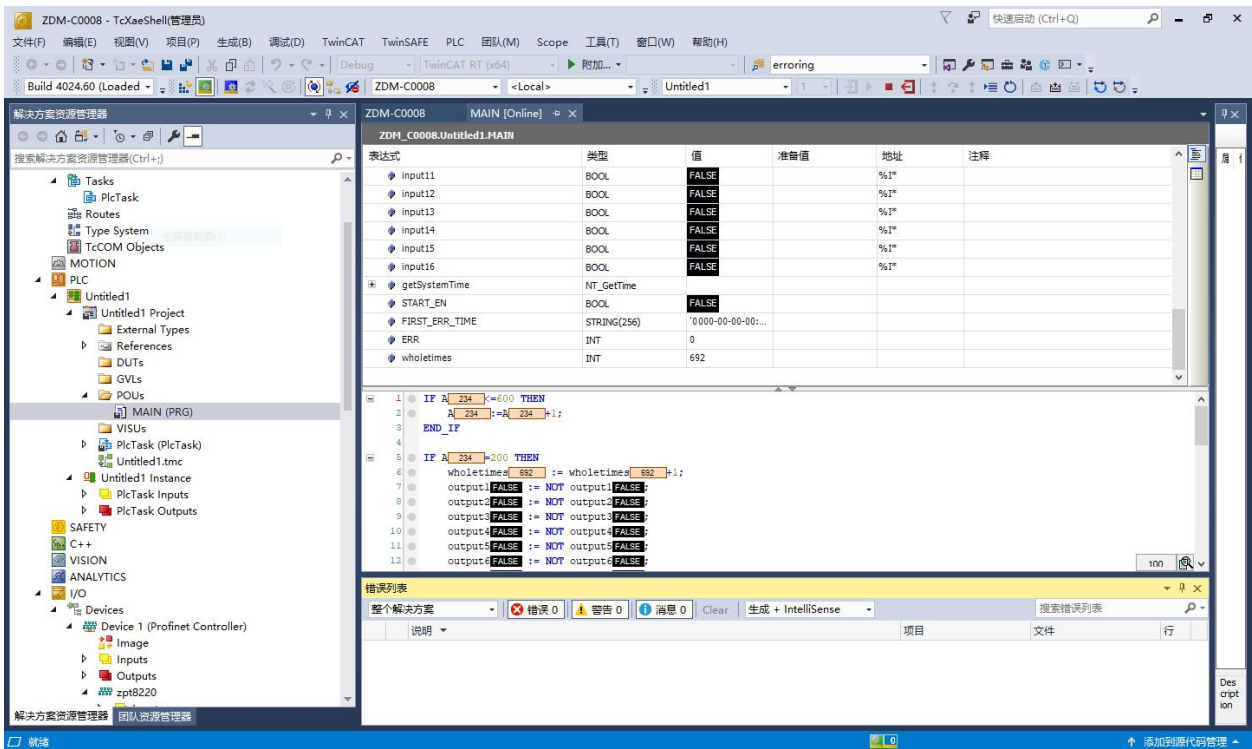
图 3 功能测试截图
