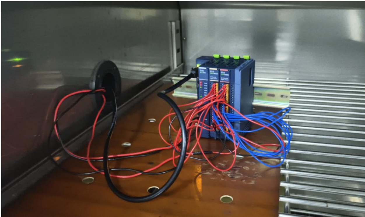
图 4 样机测试环境图
