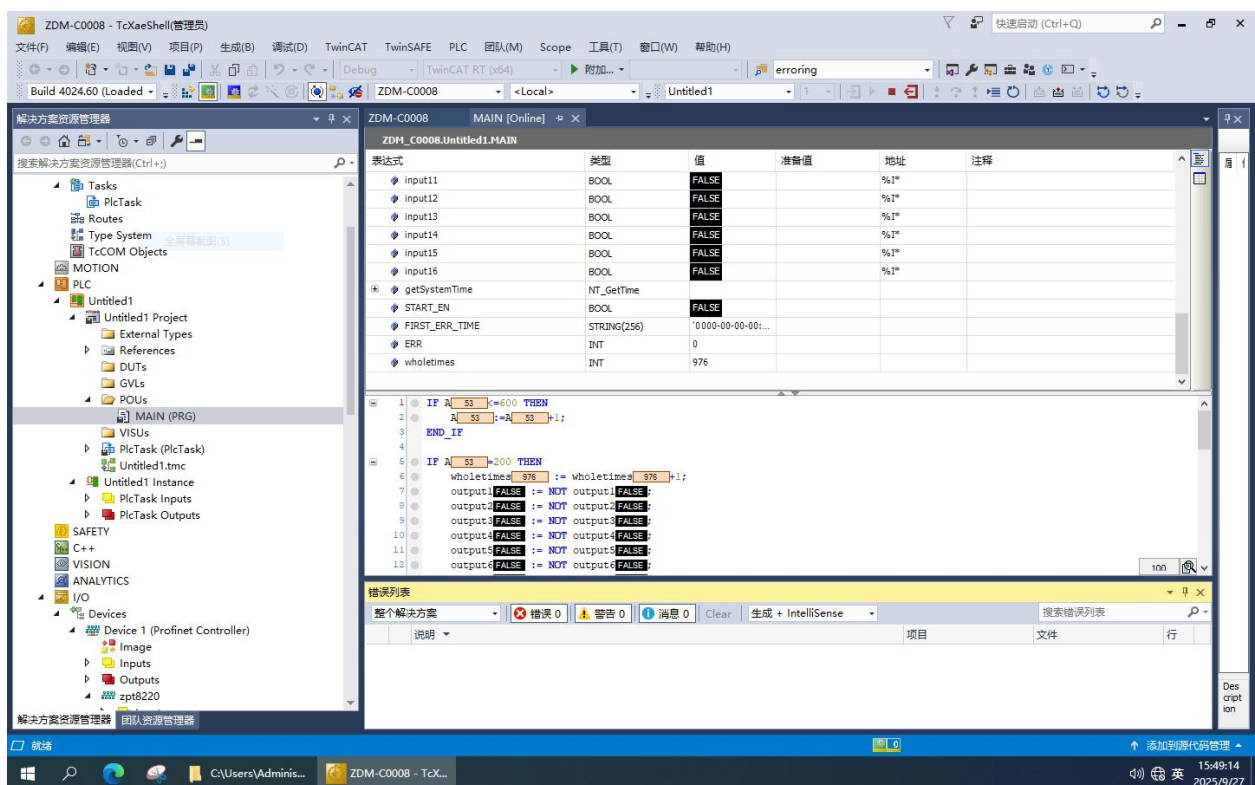
图 11 样机在低温试验时第三次启动运行检查功能正常（36VDC 供电）
