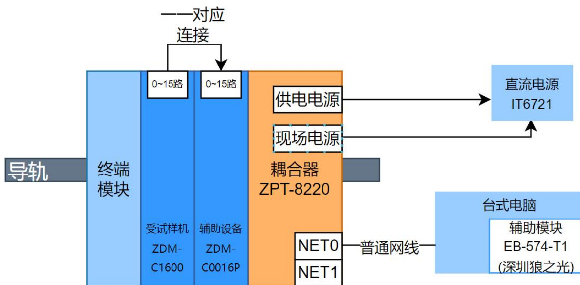
图 1 试验配置图
