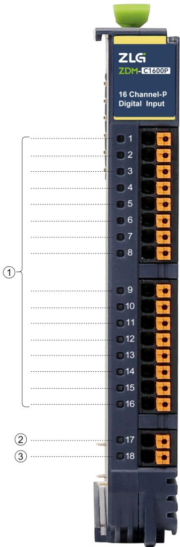
图 2.2 指示灯面板
