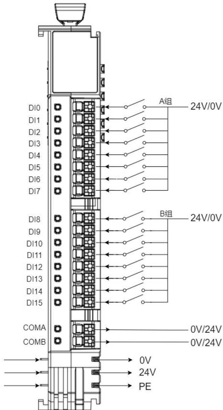
图 3.1 ZDM-C1600 模块接线图
