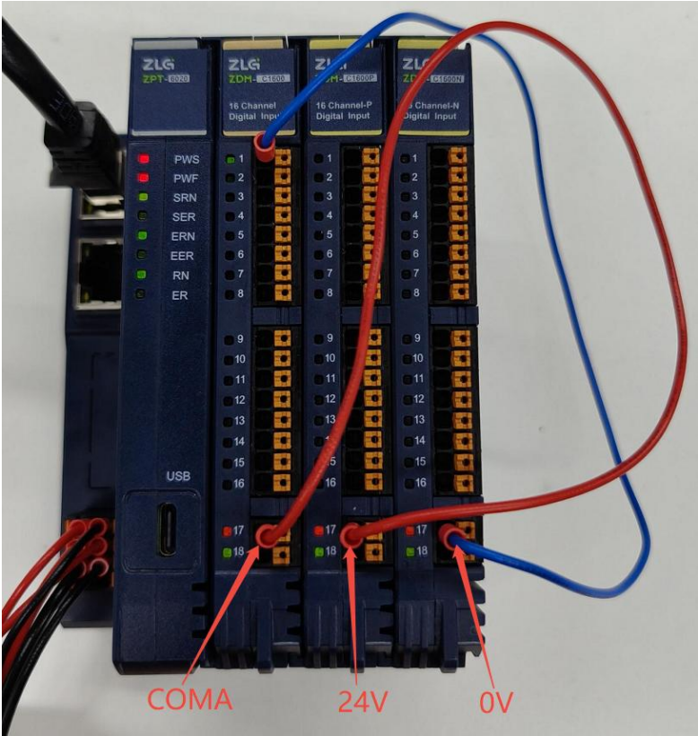
图 5.3 通道 1 输入 0V
