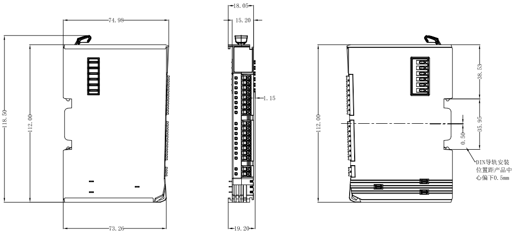
图 4.1 ZDM-C1600 产品尺寸
