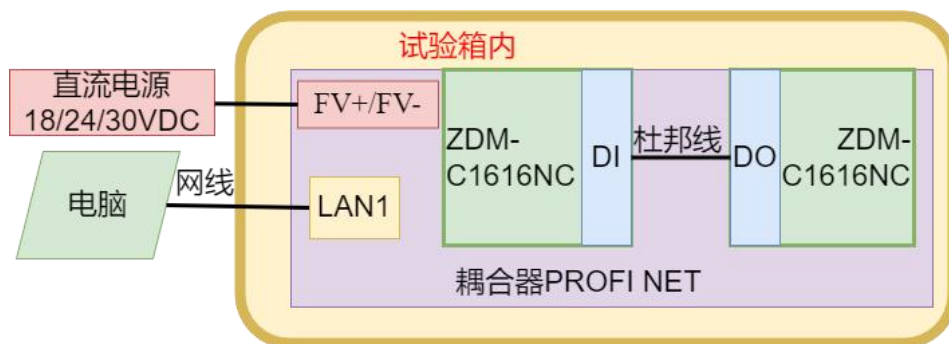
图 2 试验配置框图
