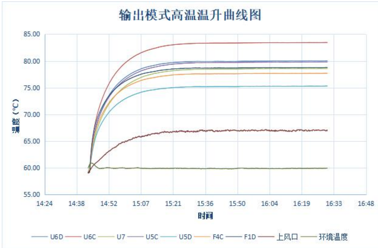
图 8 输出高温温升曲线图
