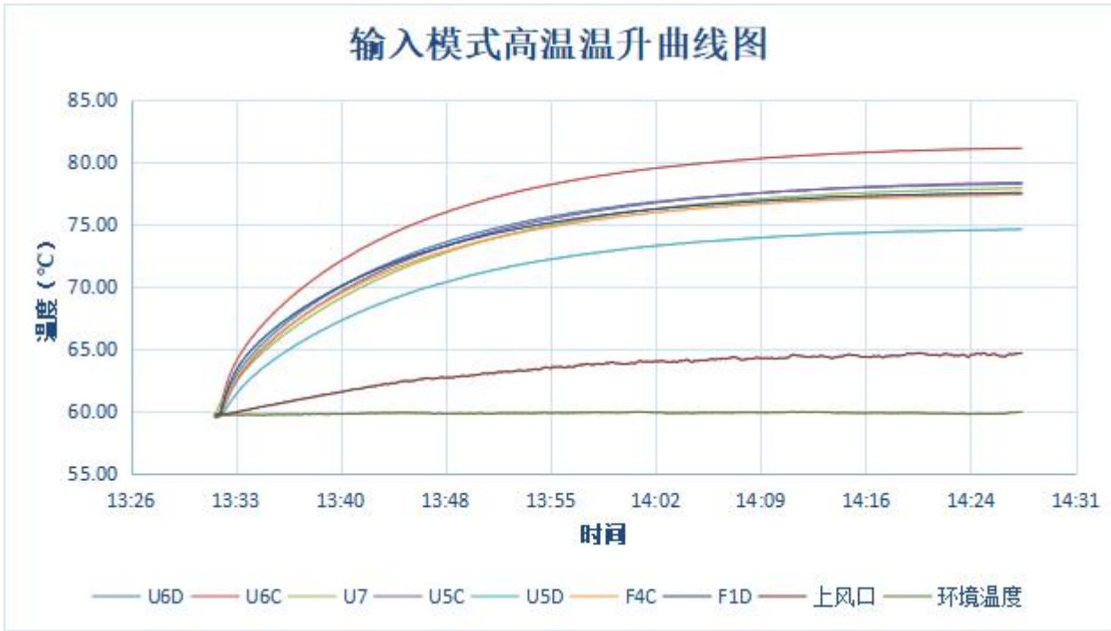
图 10 输入高温温升曲线图
