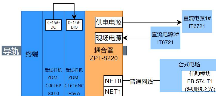
图 5 输入试验配置框图
