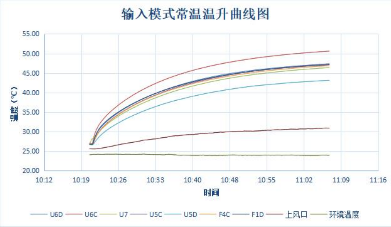
图 9 输入常温温升曲线图
