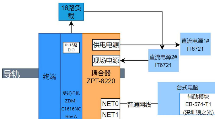
图 4 输出试验配置框图
