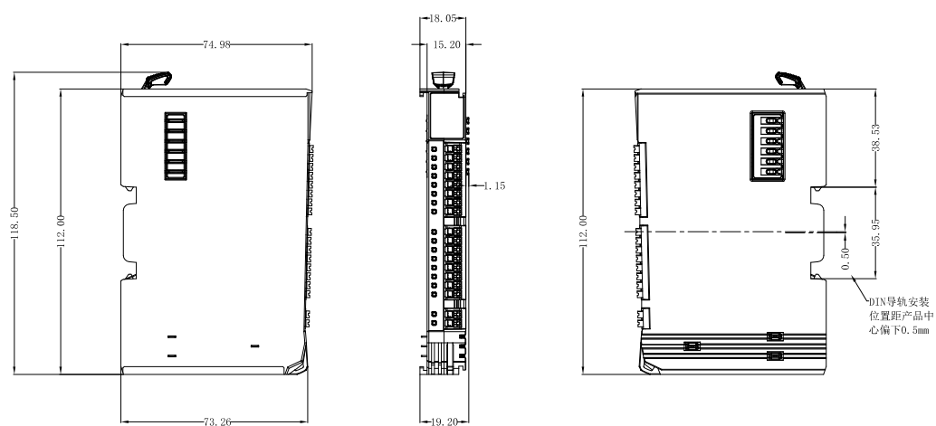
图 4.1 ZDM-C1616NC 产品尺寸
