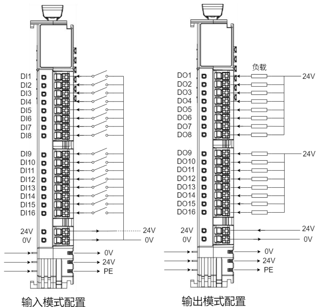
图 3.1 ZDM-C1616NC 模块接线图
