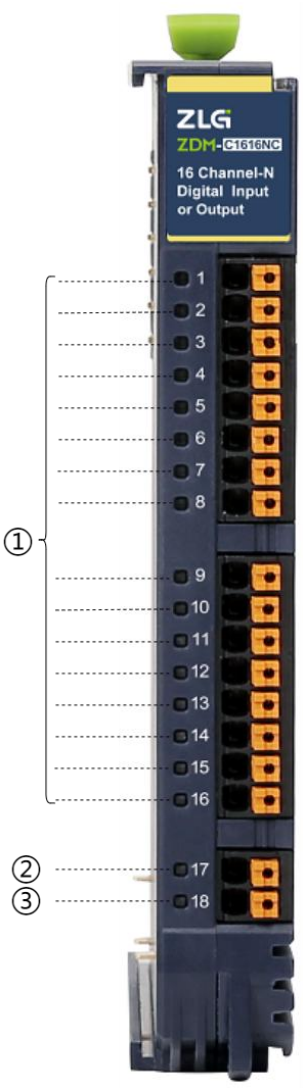
图 2.2 指示灯面板
