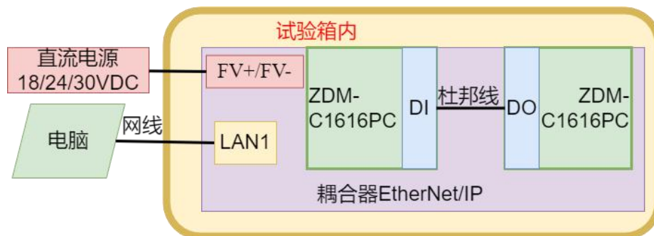
图 2 试验配置框图
