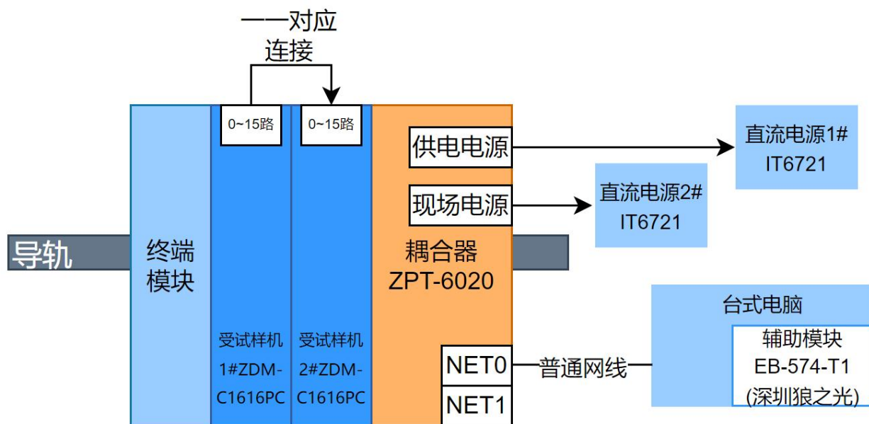
图 1 试验配置示意图
