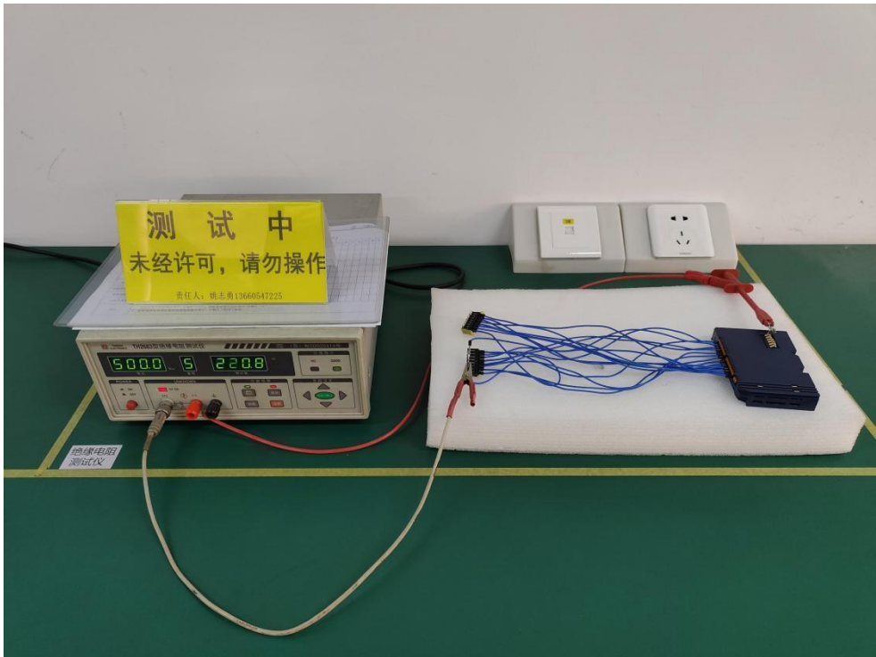
图 1 绝缘电阻试验
