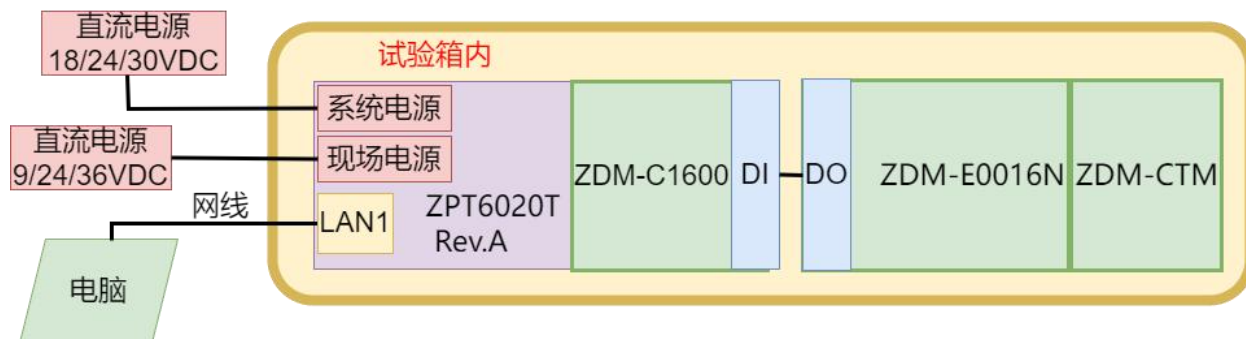
图 2 试验配置框图
