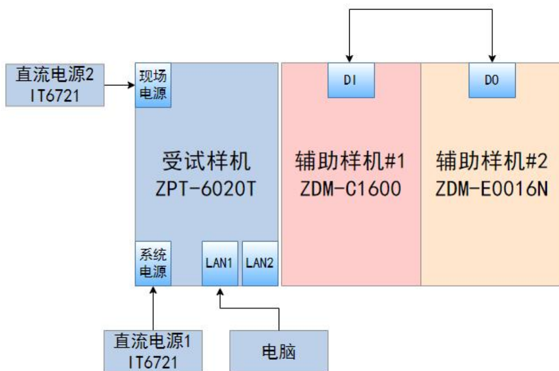
图 1 试验配置示意图
