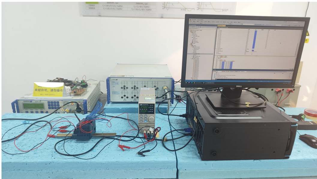
图 4 浪涌试验现场配置图
