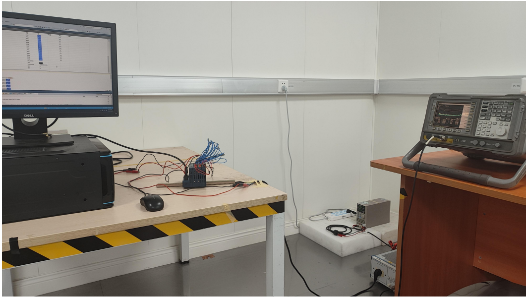
图 6 传导骚扰试验现场配置图
