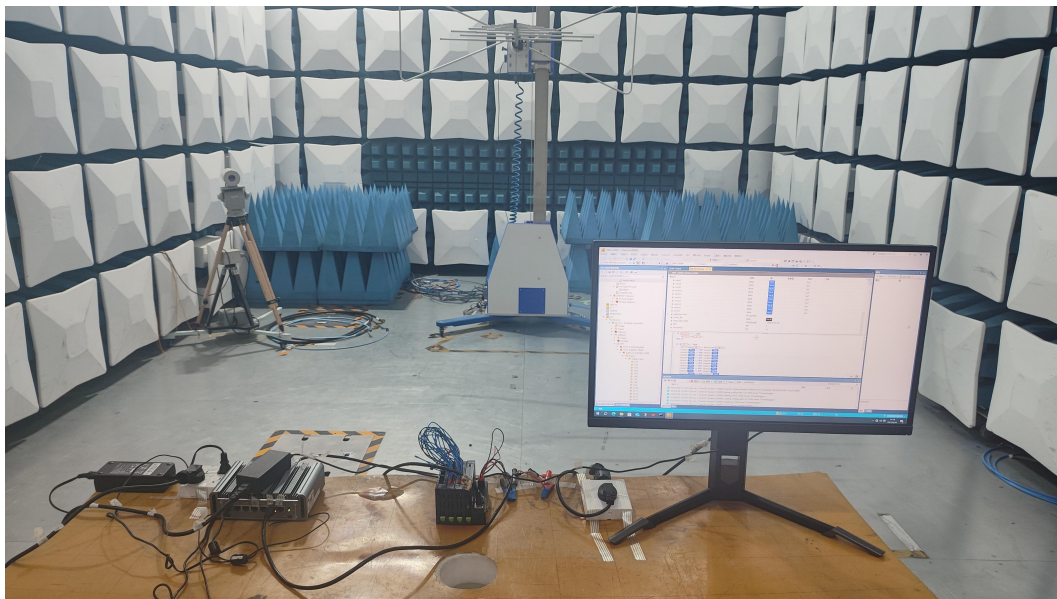
图 7 辐射骚扰试验配置
