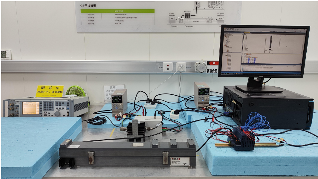
图 5 CS 试验现场配置图
