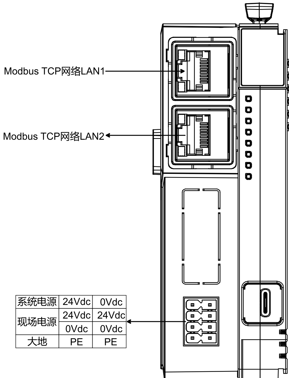
图 3.1 ZPT-6020T 模块接线说明
