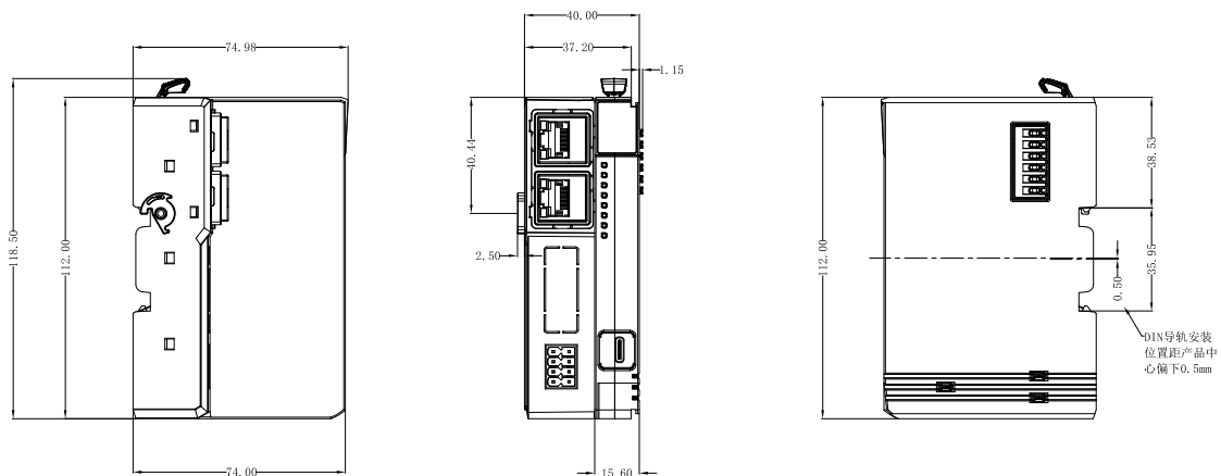
图 4.1 ZPT-6020T 产品尺寸
