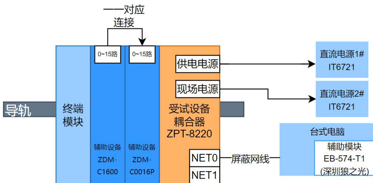
图 1 试验配置图
