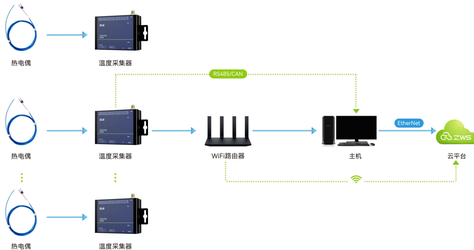
图 4.1 多设备级联网络示意图
