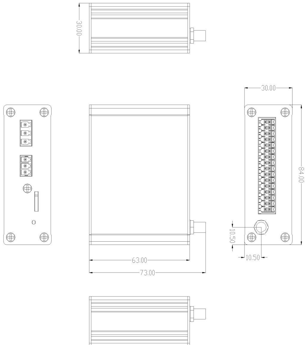
图 1.2 ZAD2116 尺寸图
