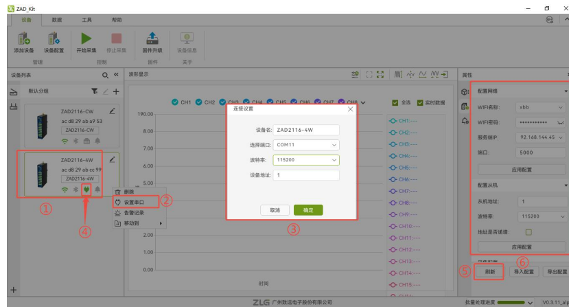
图 4.19 通过 RS-485 配置设备参数
