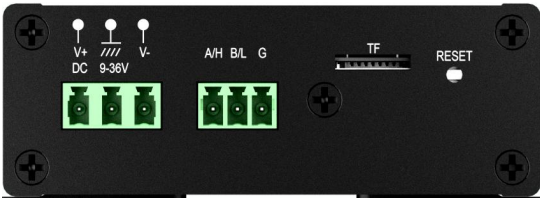
图 3.2 底部接口示意图
