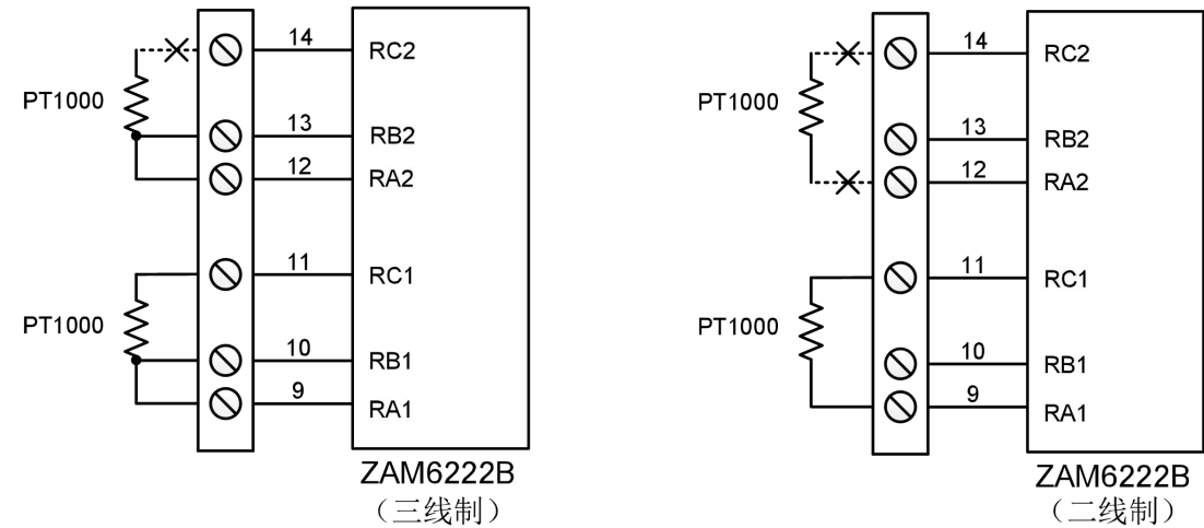
图 3.10 ZAM6222B 断线情况图示
