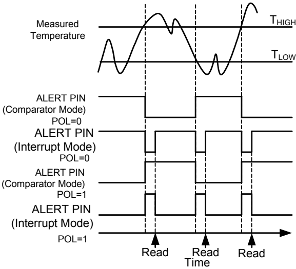
图 3.9 ALERT 信号输出状态设置图示
