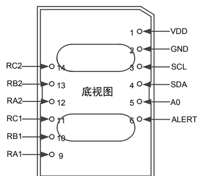
图 2.2 ZAM6222B 引脚底视图
