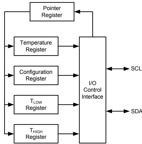
图 3.8 寄存器结构示意图
