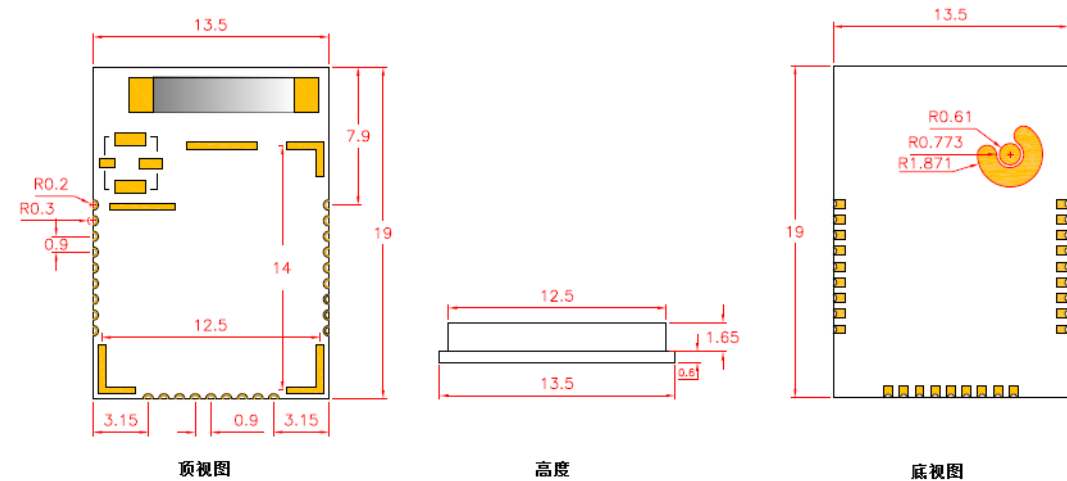
图 2.3 AW5161P2xx 尺寸图 (单位: mm)
