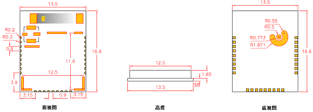
图 2.1 AW5161P0xx 尺寸图 (单位: mm)
