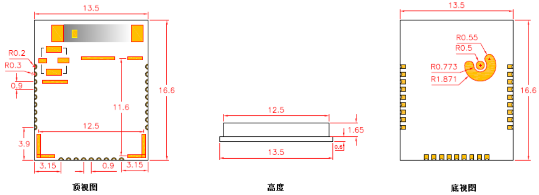
图 2.2 AW5169P1xx 尺寸图 (单位: mm)
