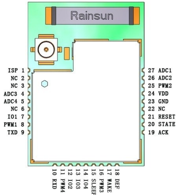
图 3.1 引脚分布图
