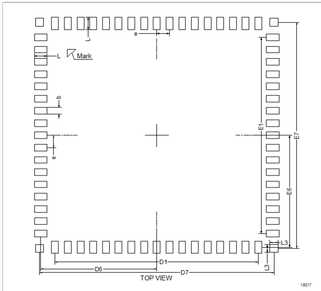
图 20. 封装参考图
