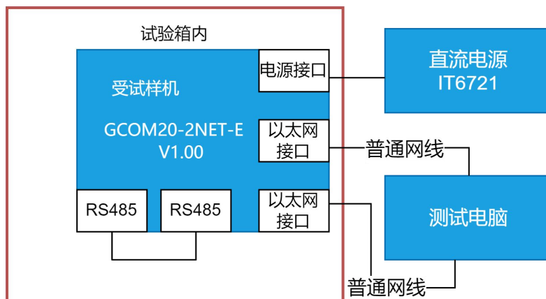
图 2 试验配置框图
