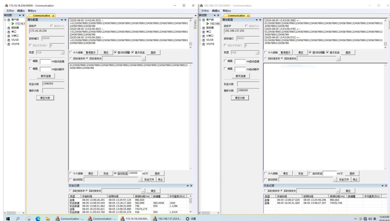
图 8 样机在低温试验时第二次启动运行检查功能正常(36V)
