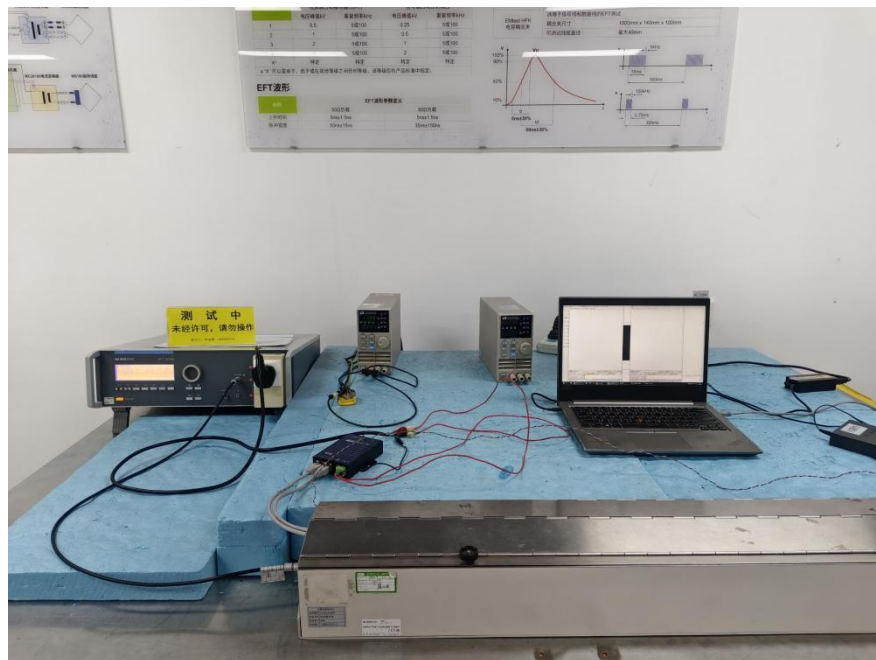
图 6 EFT/B 试验配置
