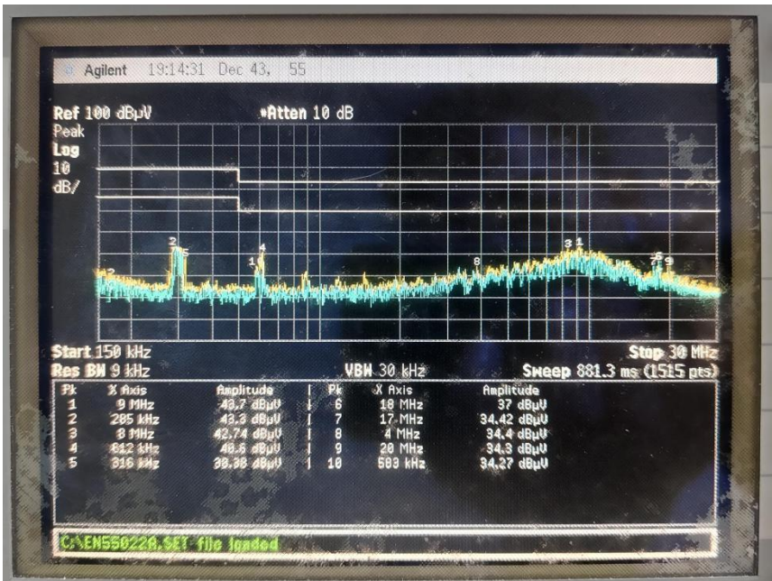
EUT-N 线
