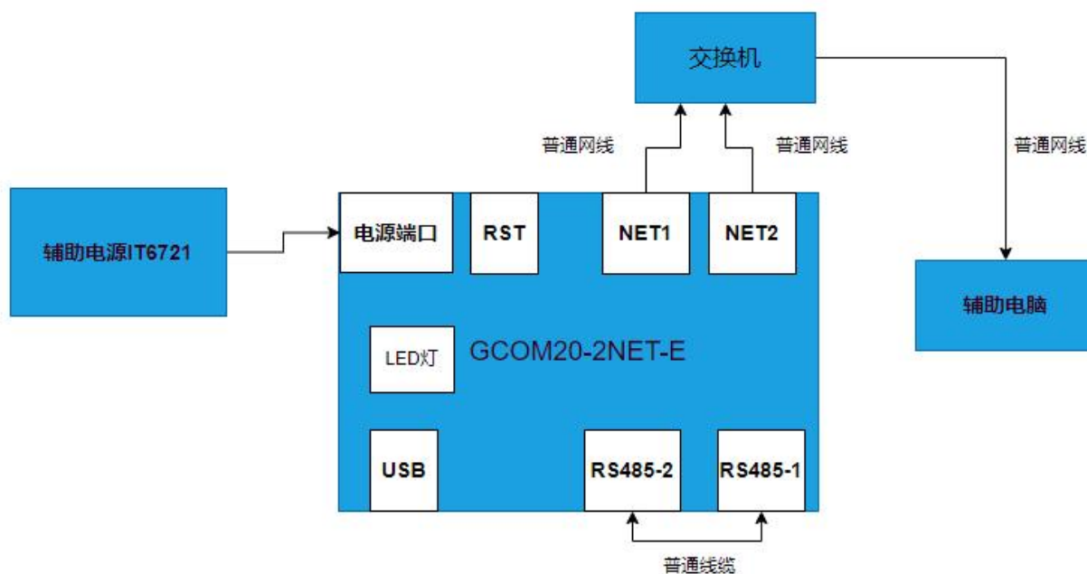
图 1 试验配置示意图
