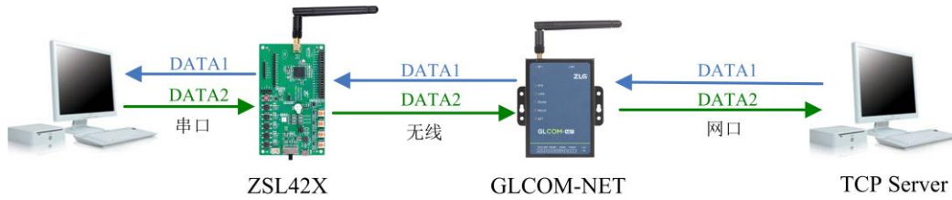
图 3.11 无线与 TCP Client 透传应用示意图
