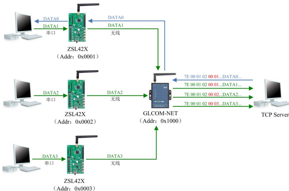
图 4.45 无线与 TCP Client 一对多透传应用示意图
