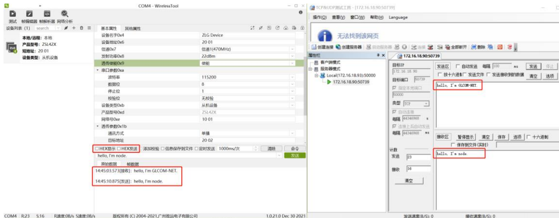
图 3.20 无线节点与 TCP 服务器透明数据收发
