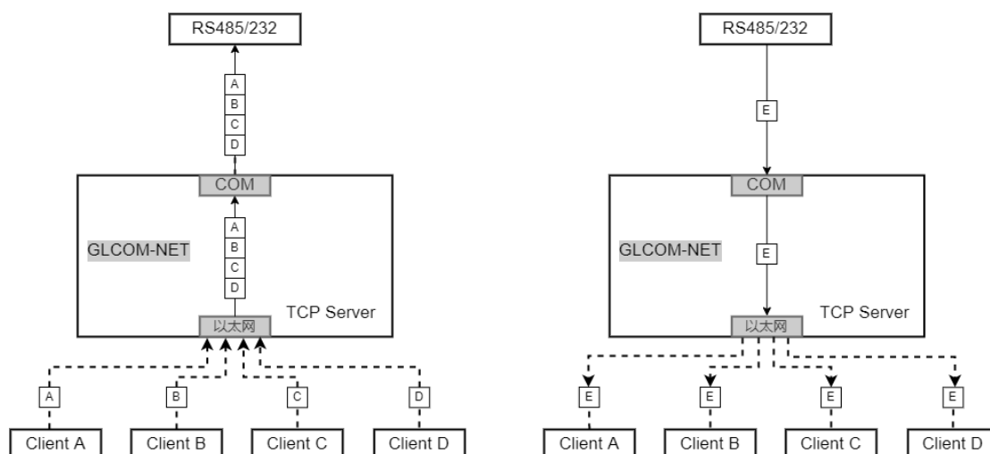
图 4.30 串口转 TCP Server 示意图
