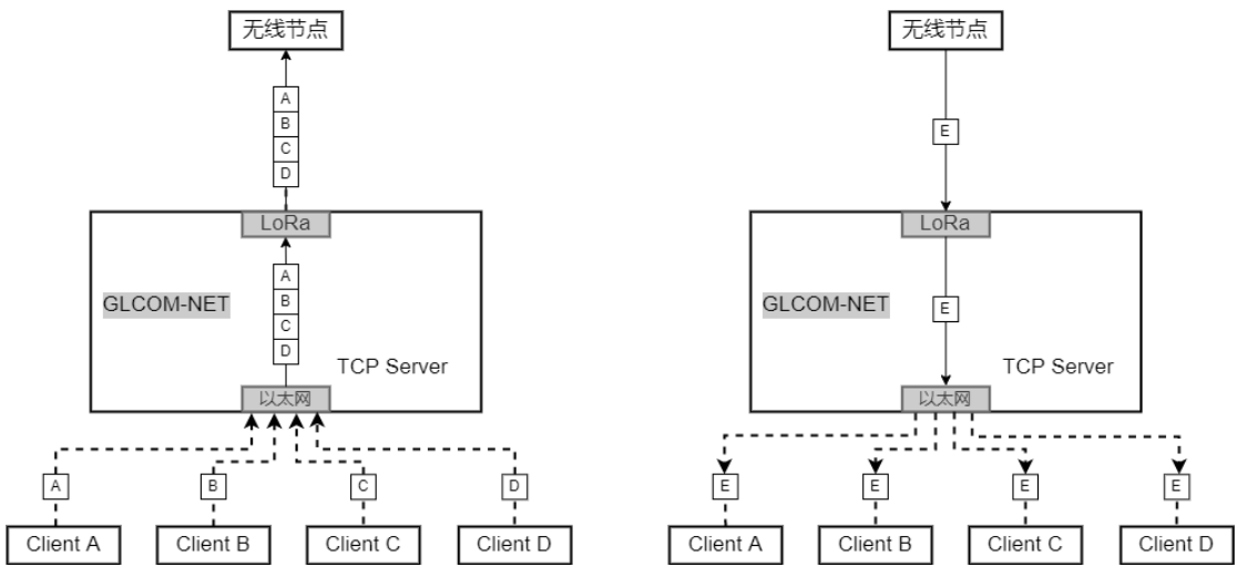
图 4.1 无线转 TCP Server 示意图
