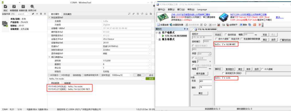
图 4.6 无线节点与 TCP Client 数据收发
