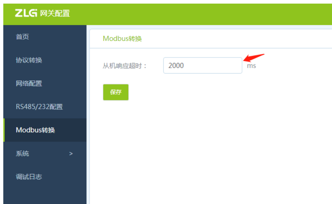
图 4.39 设置从机响应超时
