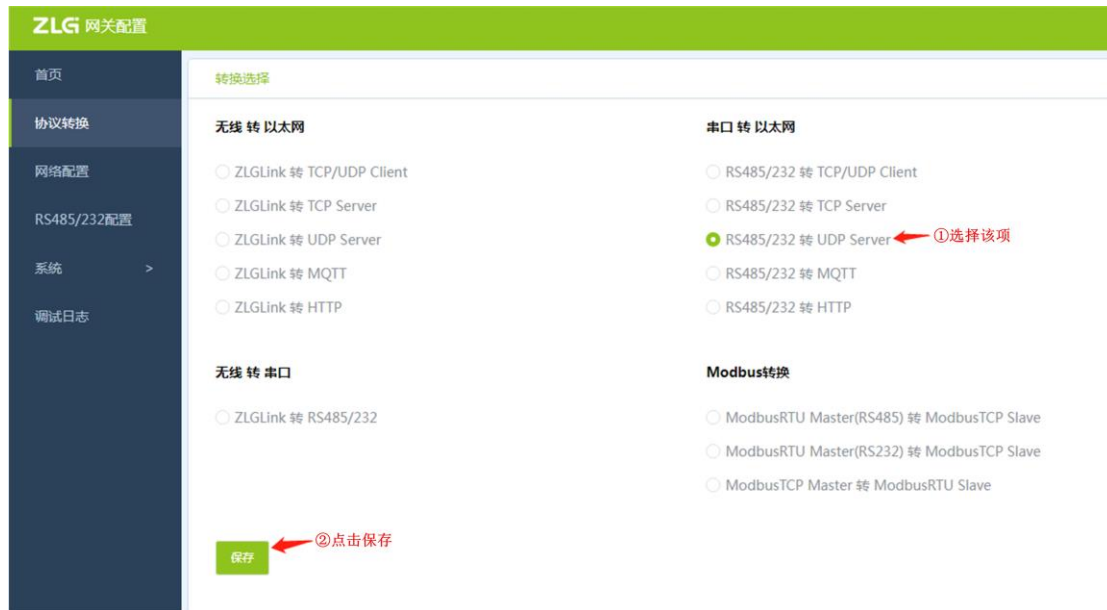
图 4.32 选择 RS485/232 转 UDP Server
