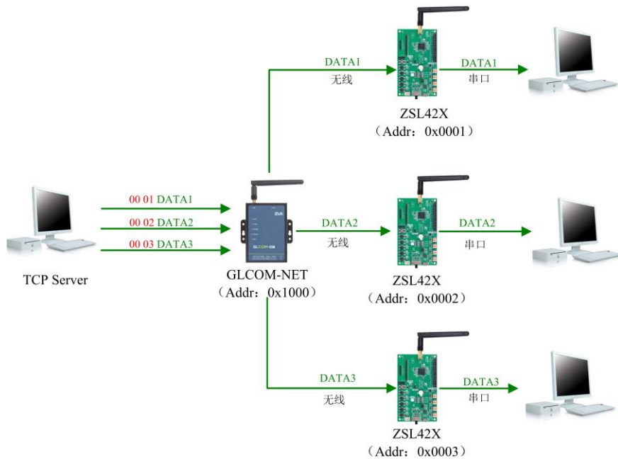
图 5.22 发送透传数据头包含目标地址
