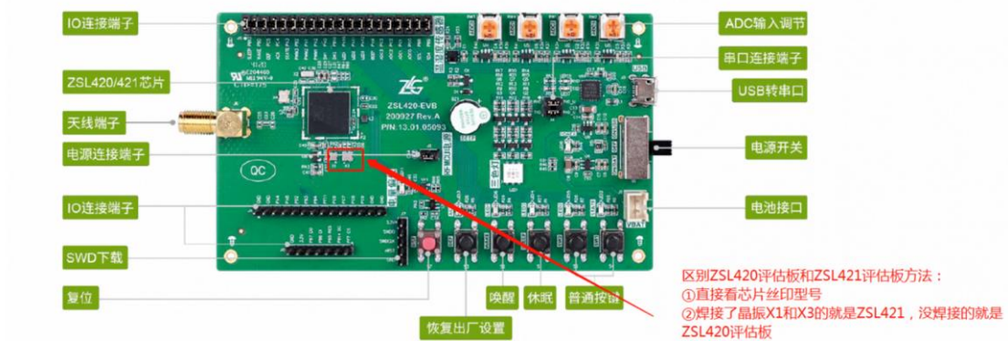
图 3.2 ZSL42x 评估板
