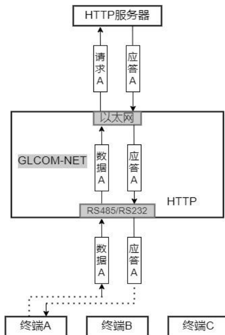
图 4.35 串口转 HTTP 示意图
