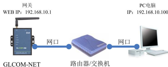
图 3.4 通过路由器连接
