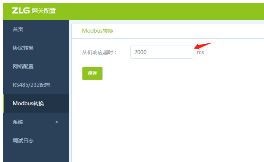
图 4.41 设置从机响应超时
