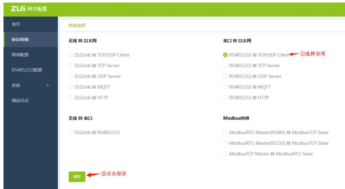
图 4.29 选择 RS485/232 转 TCP/UDP Client
