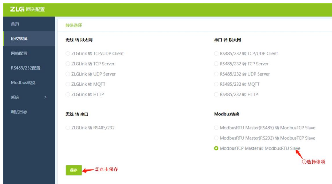
图 4.43 选择 ModbusTCP Master 转 ModbusRTU Slave
