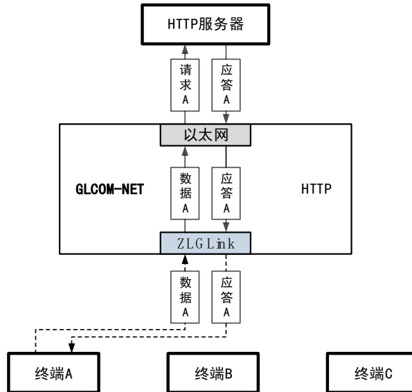
图 4.17 无线转 HTTP 通信示意图
