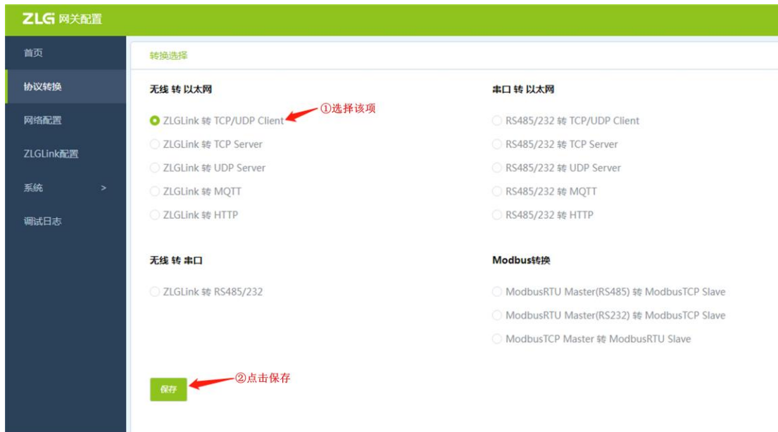
图 3.12 选择 ZLGLink 转 TCP/UDP Client
