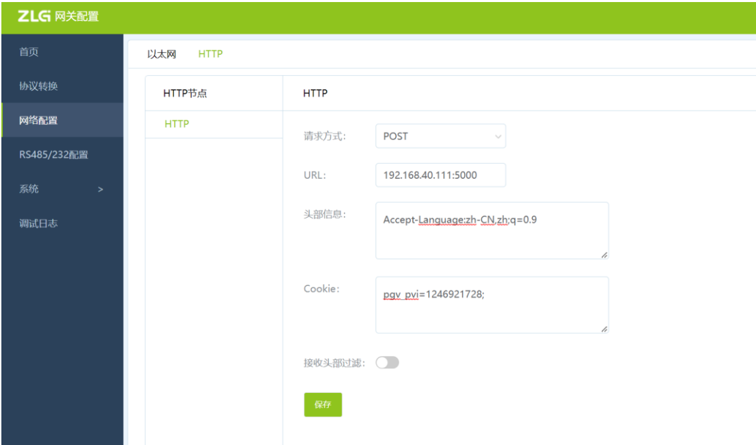
图 4.21 HTTP 配置示例 2
