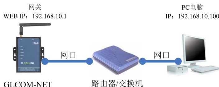
图 5.2 通过路由器连接
