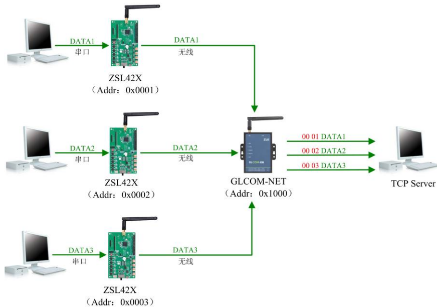
图 5.23 接收透传数据头包含源地址
