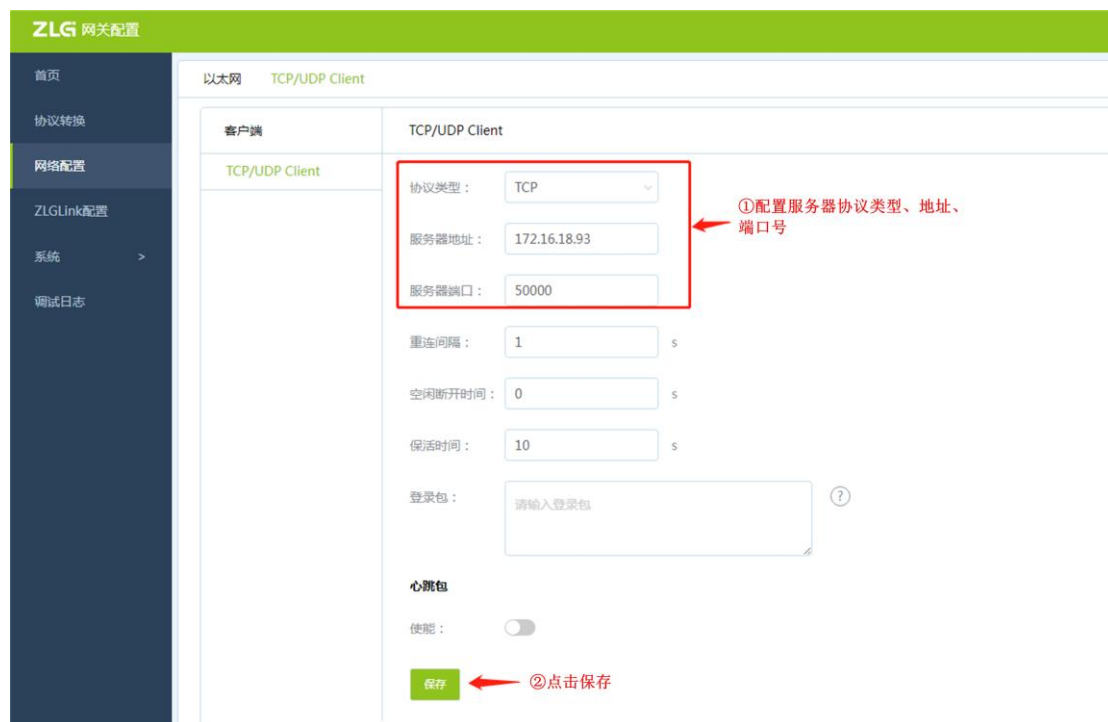
图 3.14 配置 TCP/UDP Client 参数
