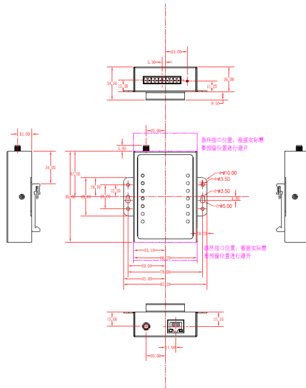
图 2.4 带轨道安装工具的外观尺寸
