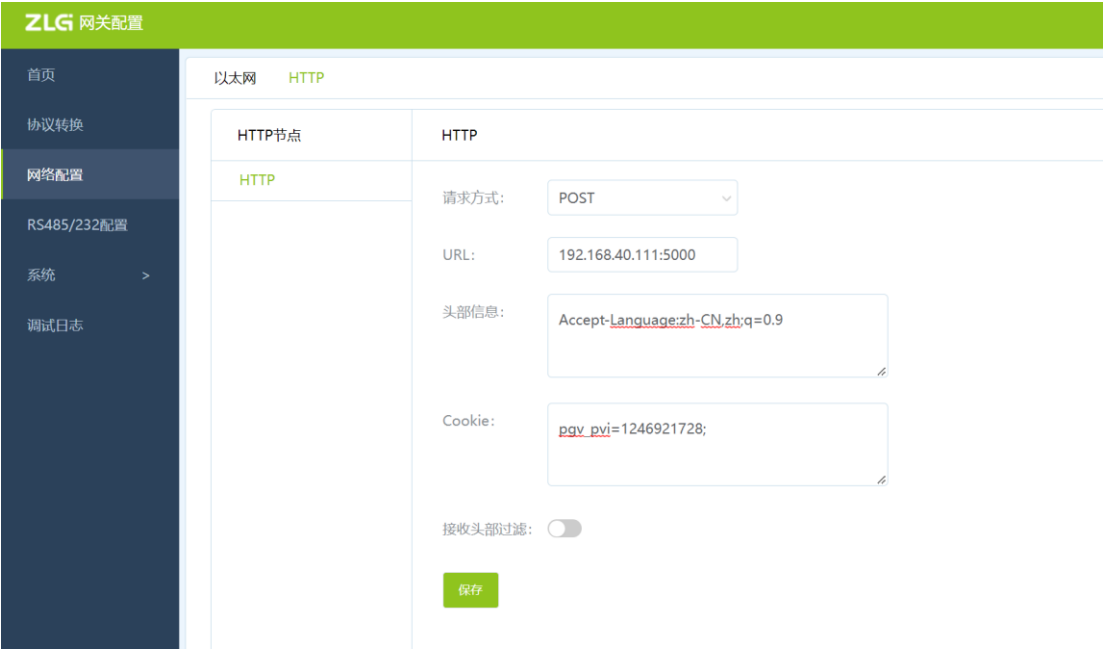
图 5.20 HTTP 配置示例 2
