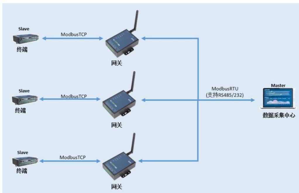
图 4.37 ModbusRTU Master 转 ModbusTCP Slave
