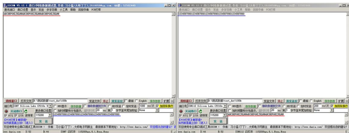
图 4.28 无线与 RS485/232 透明数据收发
