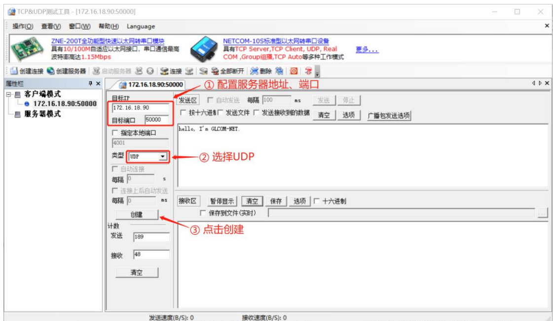
图 4.15 UDP Client 配置
