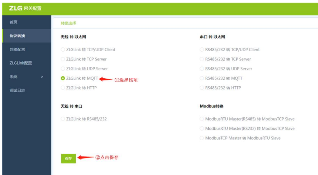
图 4.8 选择 ZLGLink 转 MQTT
