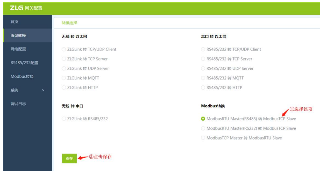
图 4.38 选择 ModbusRTU Master(RS485) 转 ModbusTCP Slave
