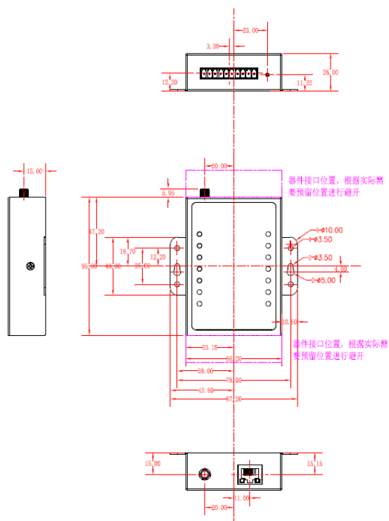
图 2.3 不带轨道安装工具的外观尺寸
