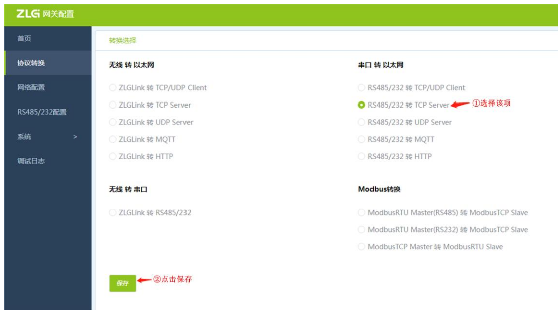
图 4.31 选择 RS485/232 转 TCP Server
