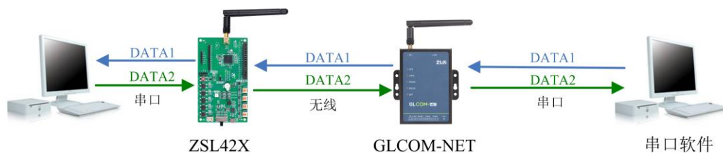
图 4.23 无线与 RS485/RS232 透传应用示意图
