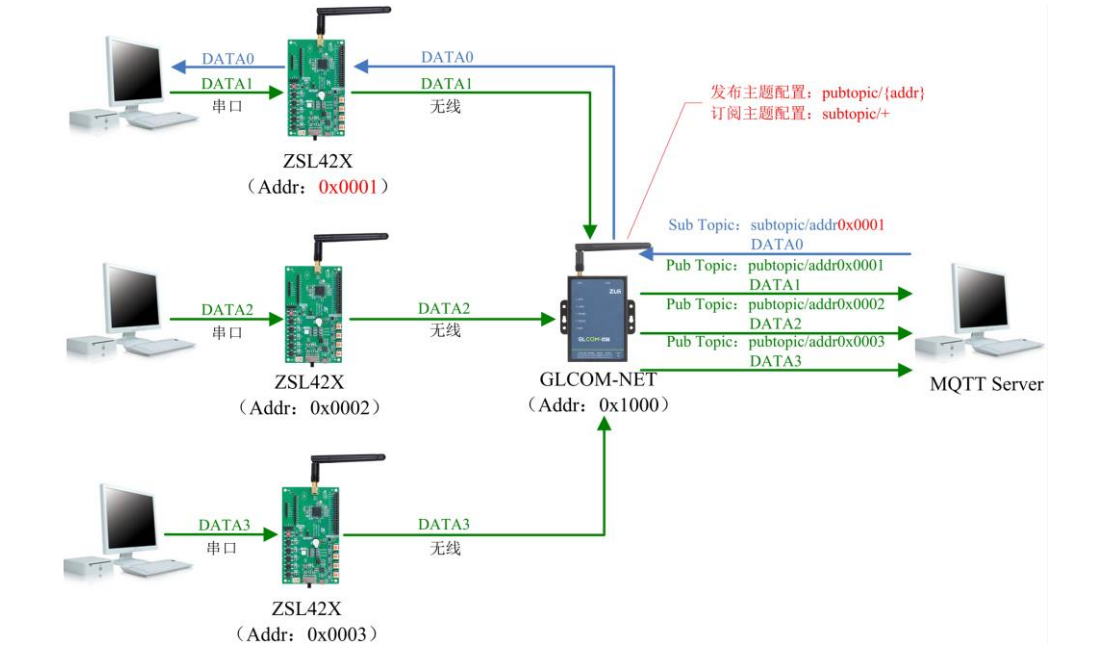
图 4.12 无线与 MQTT 一对多透传应用示意图
