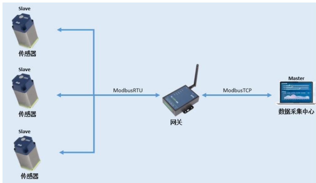
图 4.42 ModbusTCP Master 转 ModbusRTU Slave
