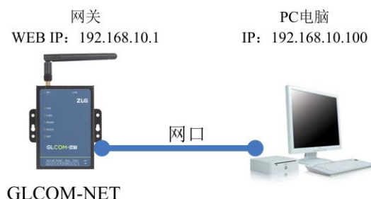
图 5.1 网关与 PC 电脑直连
