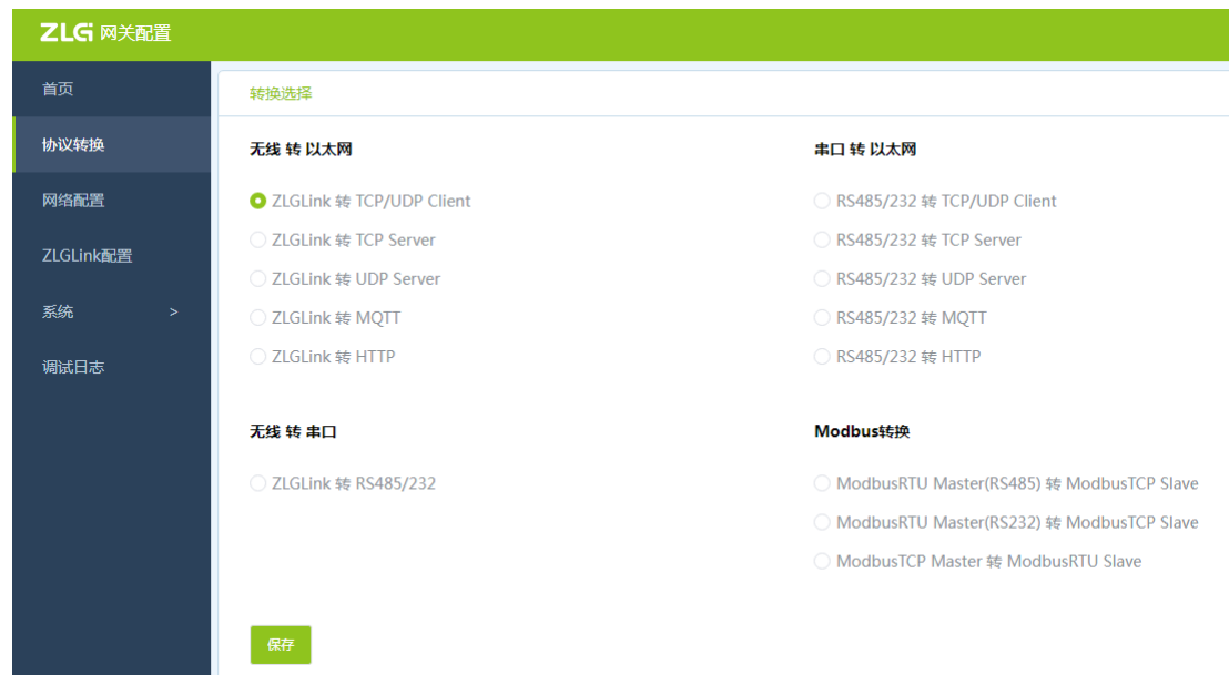
图 5.9 协议转换选择
