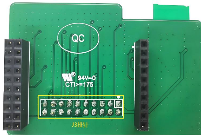
图 3.2 蓝牙模组 Pack 板反面
