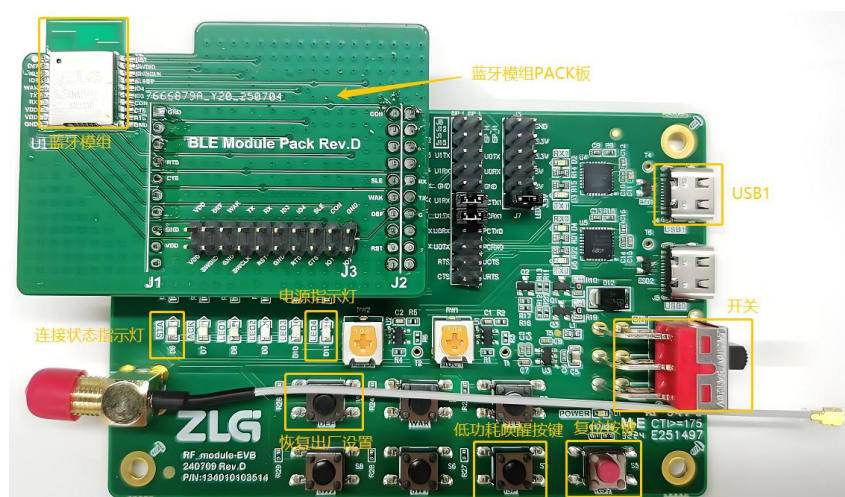
图 5.4 评估套件与蓝牙模组 Pack 板连接
