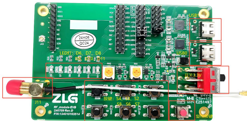
图 2.1 评估套件底板正面
