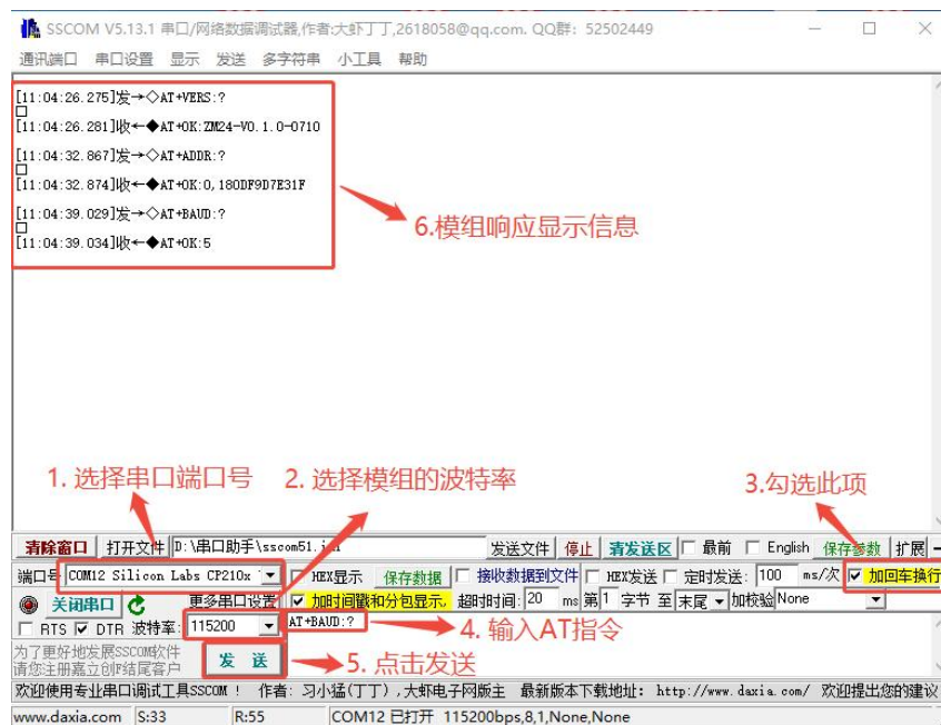
图 5.6 串口使用
