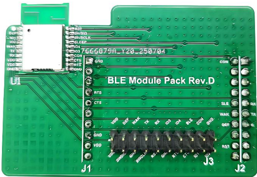
图 5.2 蓝牙模组 Pack 板
