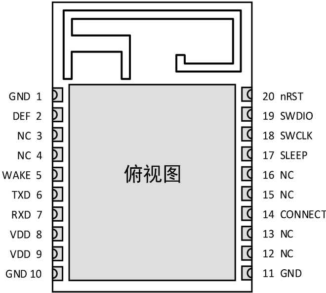
图 3.1 引脚定义
