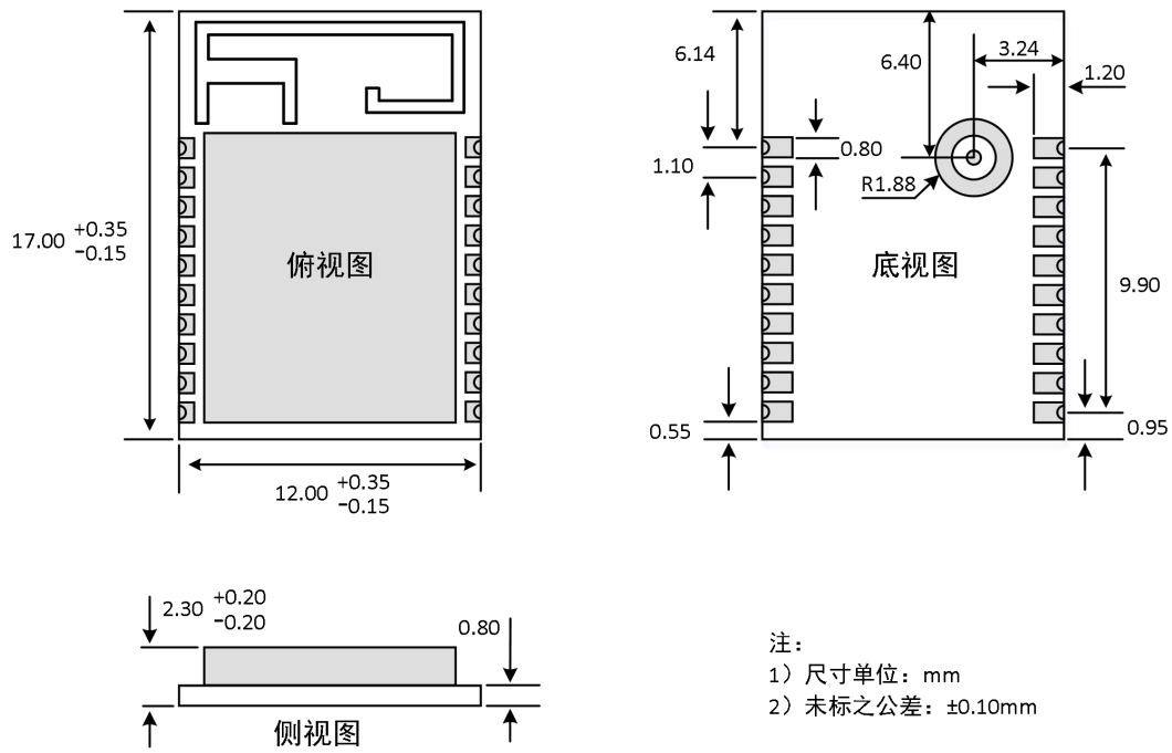
图 2.1 ZM24 系列模组尺寸图
