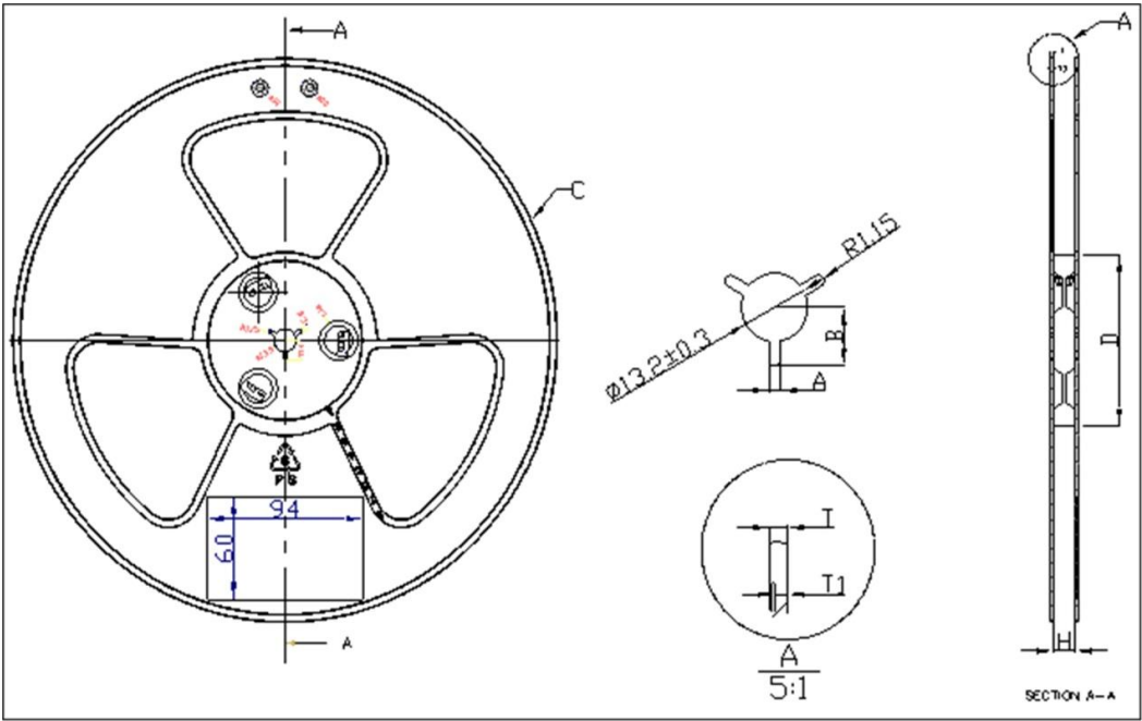
图 7.2 卷盘尺寸
