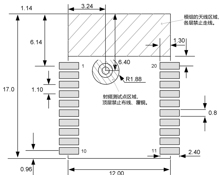
图 5.4 推荐 PCB 封装尺寸
