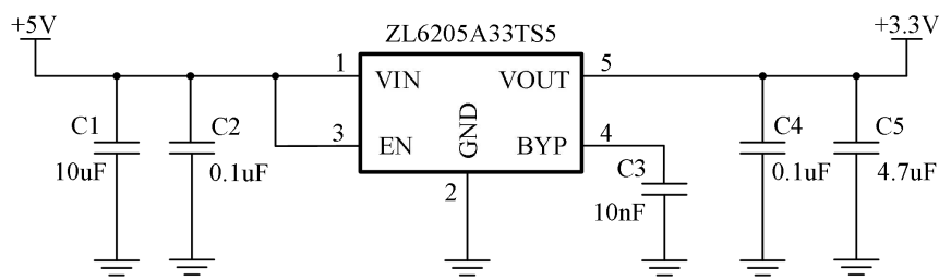
图 5.3 LDO 电源参考设计
