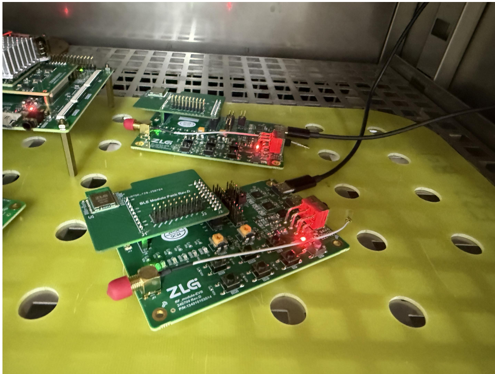
图 3 样机环境试验
