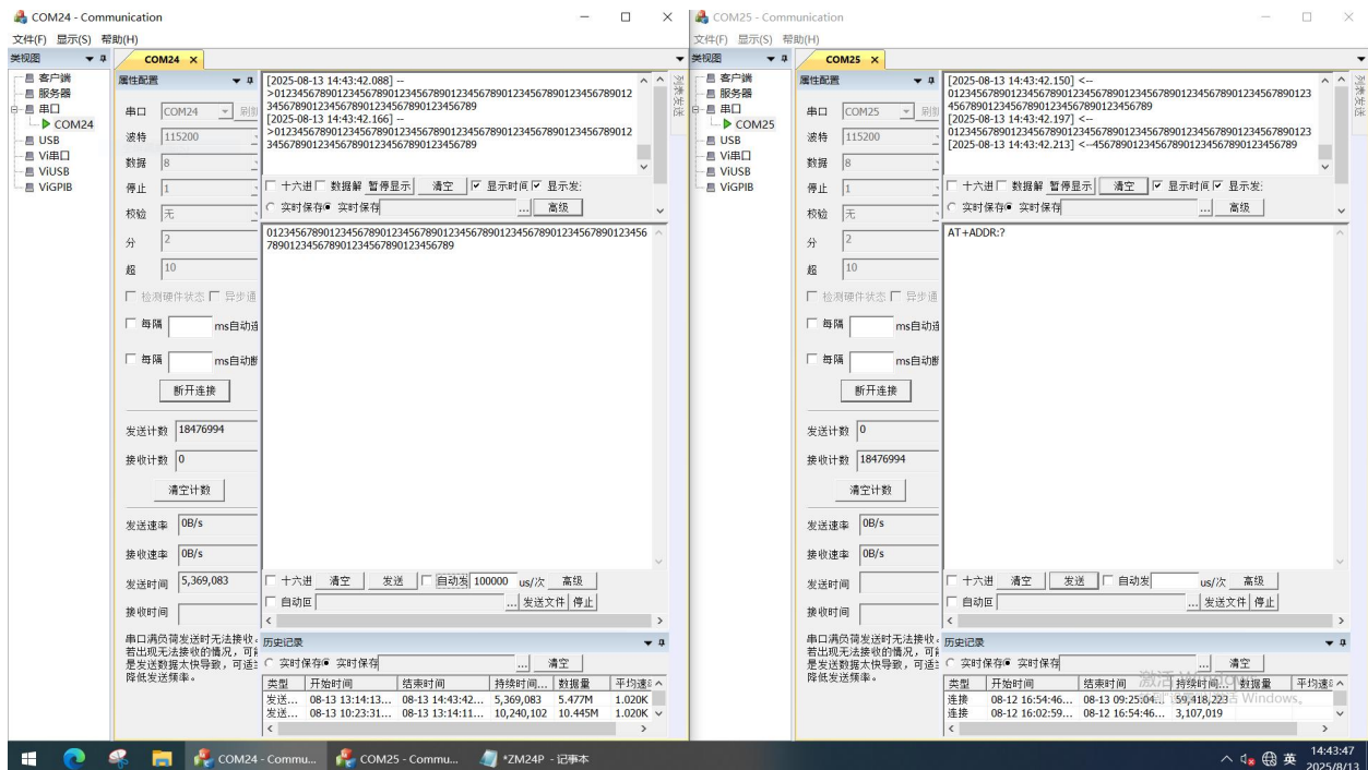
图 12 样机在高温试验时第一次启动运行检查功能正常
