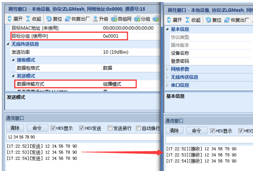
图 7.4 组播给目标分组
