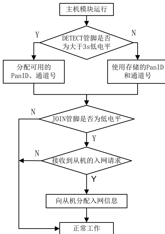
图 14.2 主机模块组网工作流程
