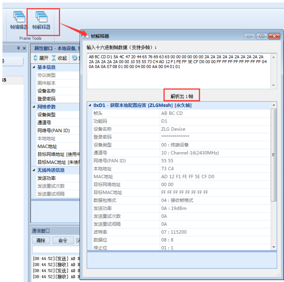
图 5.5 帧解释器功能
