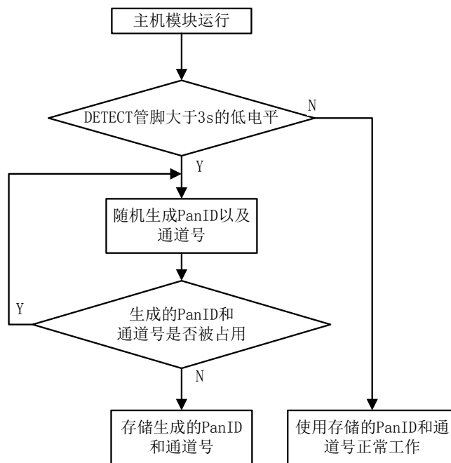
图 14.3 主机模块重获取网络参数工作流程
