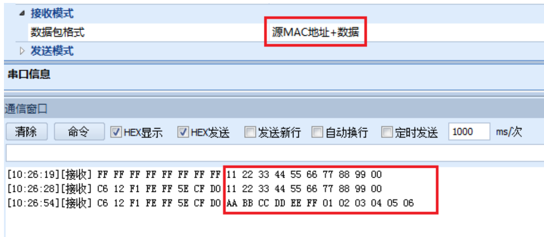
图 8.3 接收源 MAC 地址通讯
