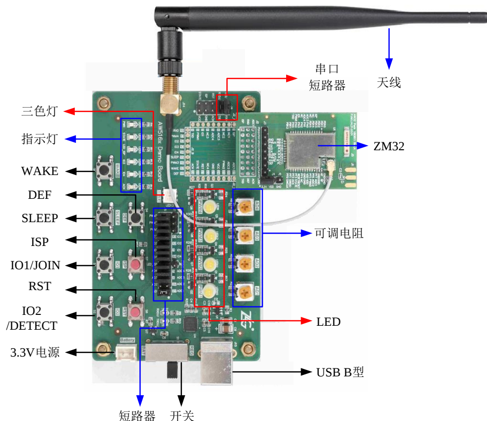
图 5.6 ZM32A Demo Board 安装图
