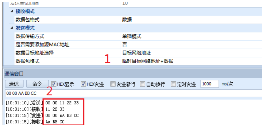
图 7.5 发送网络地址+数据
