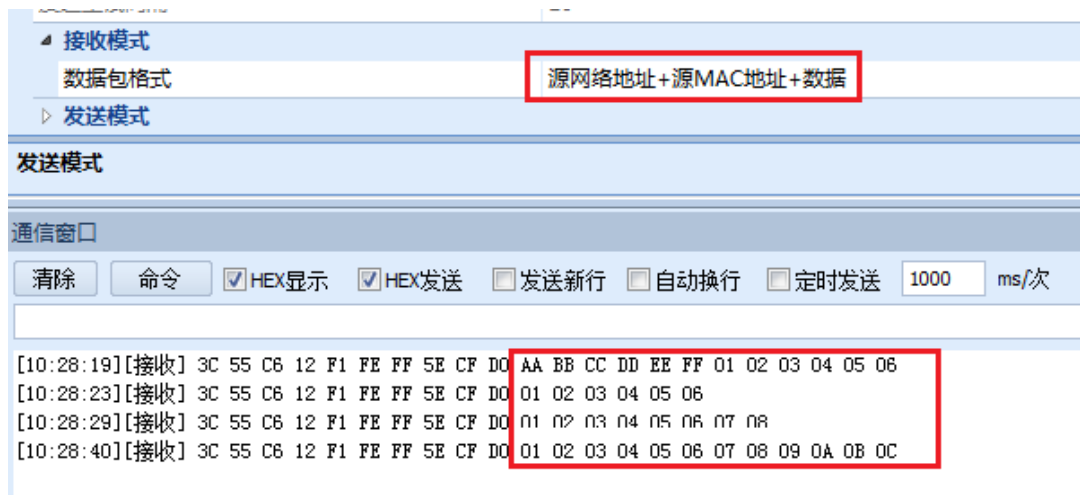
图 8.4 接收源网络地址+源 MAC 地址+数据
