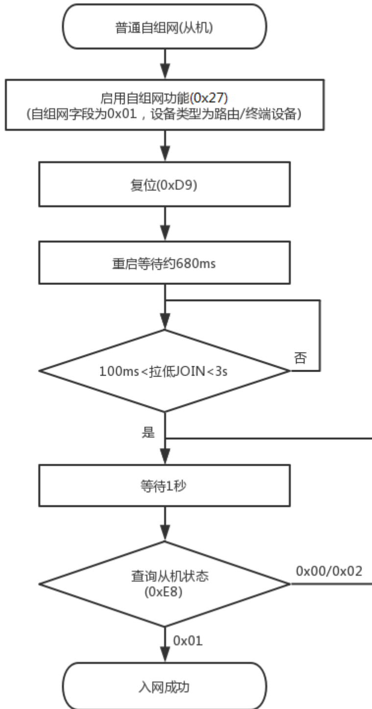
图 15.3 普通自组网-从机
