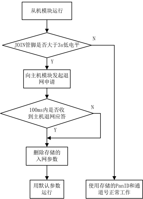
图 14.5 从机模块退网流程
