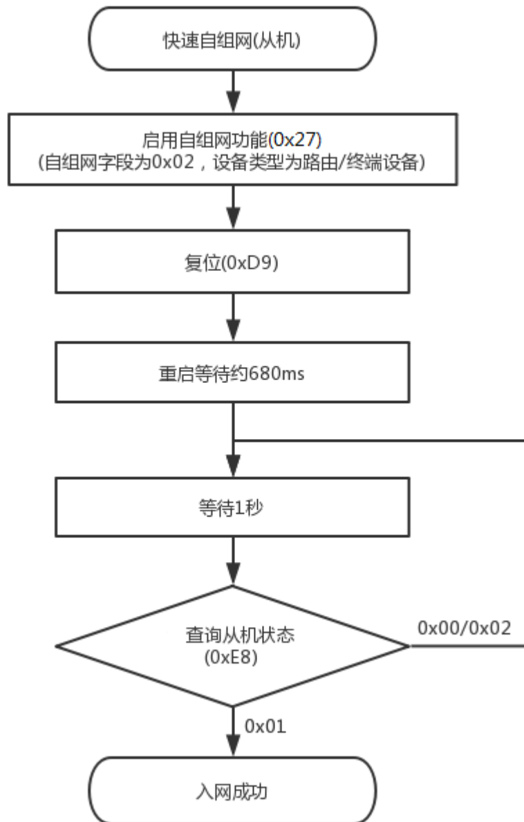
图 15.5 快速自组网-从机
