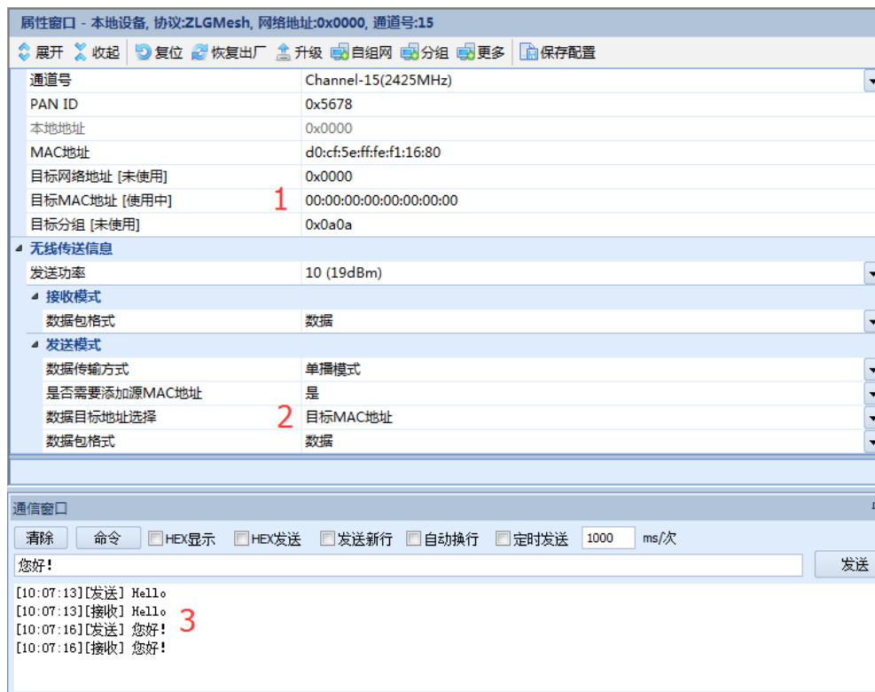
图 7.2 单播给指定目标 MAC 地址
