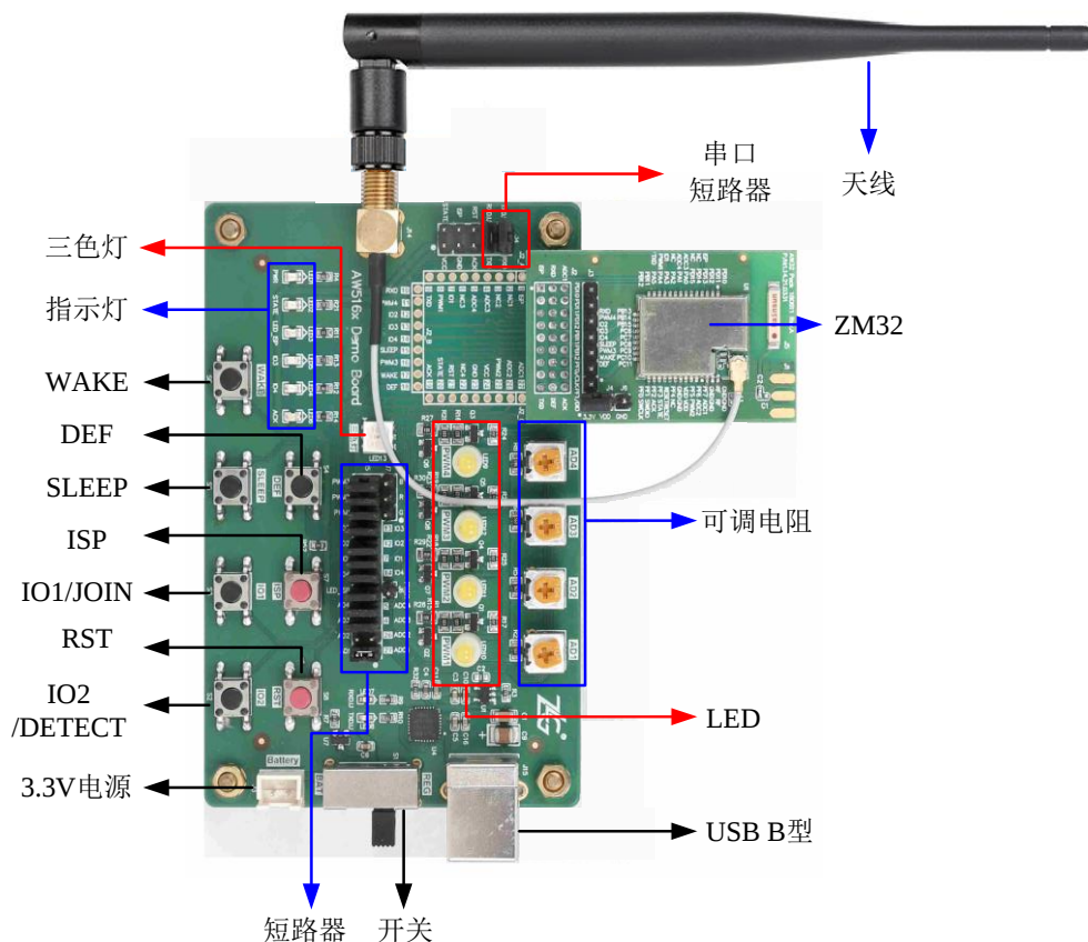
图 4.1 评估板实物图
