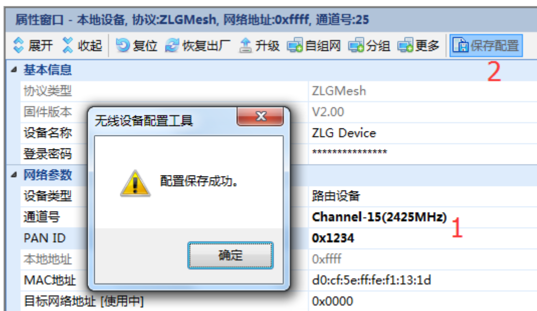
图 6.7 修改网络参数
