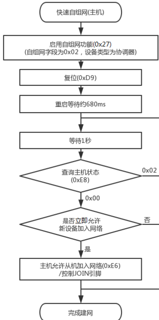
图 15.4 快速自组网-主机
