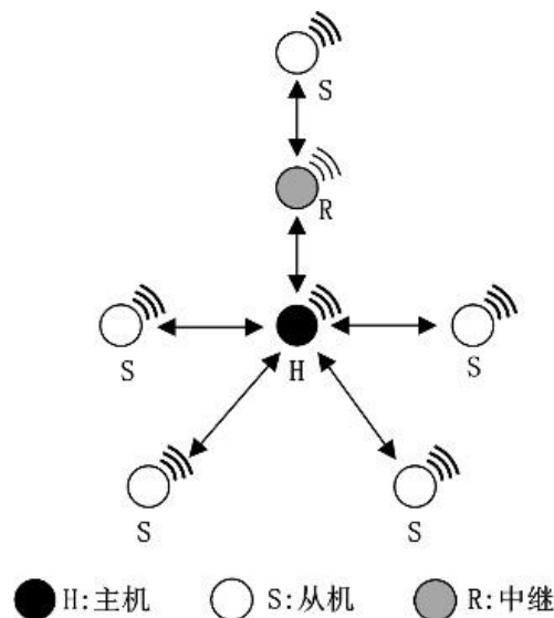
图 14.1 自组网拓扑结构
