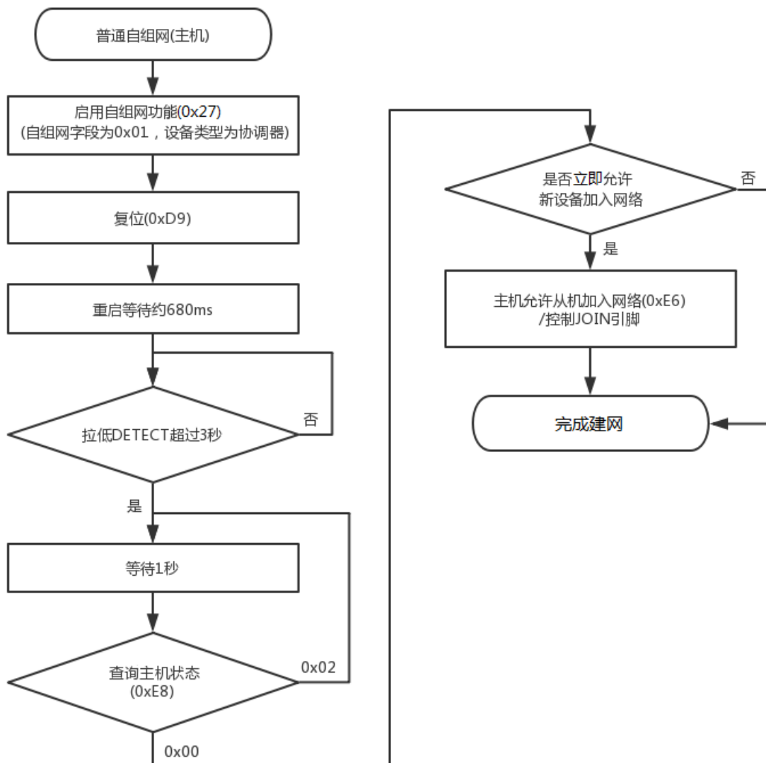
图 15.2 普通自组网-主机
