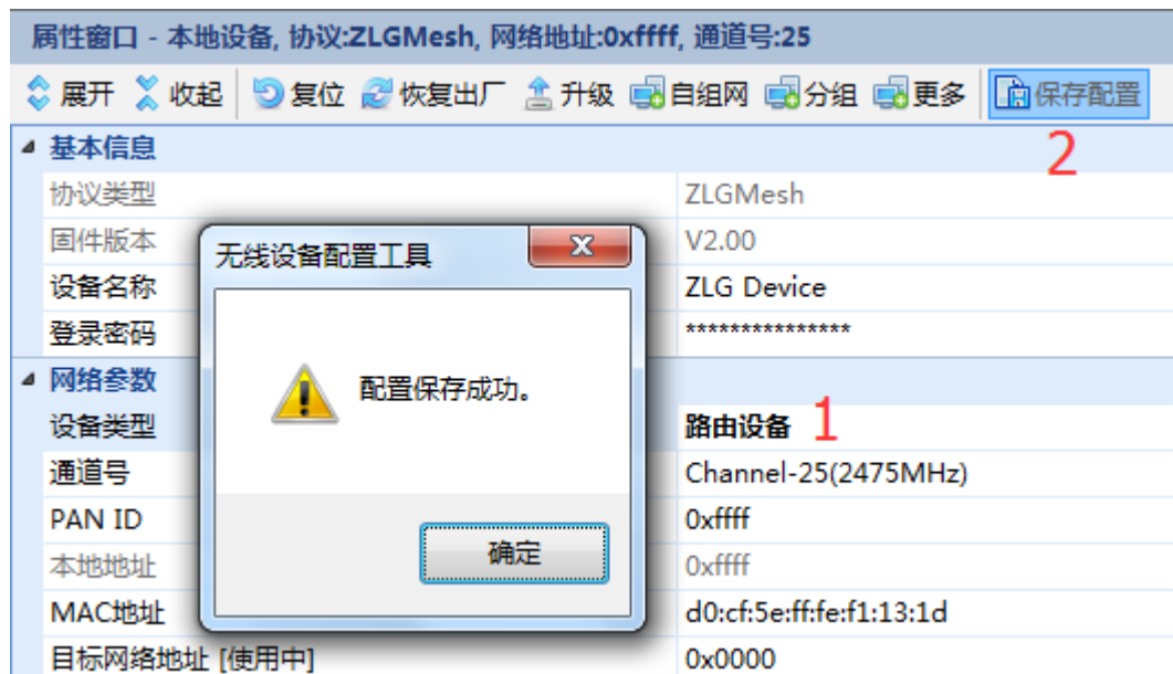
图 6.6 路由/终端设备
