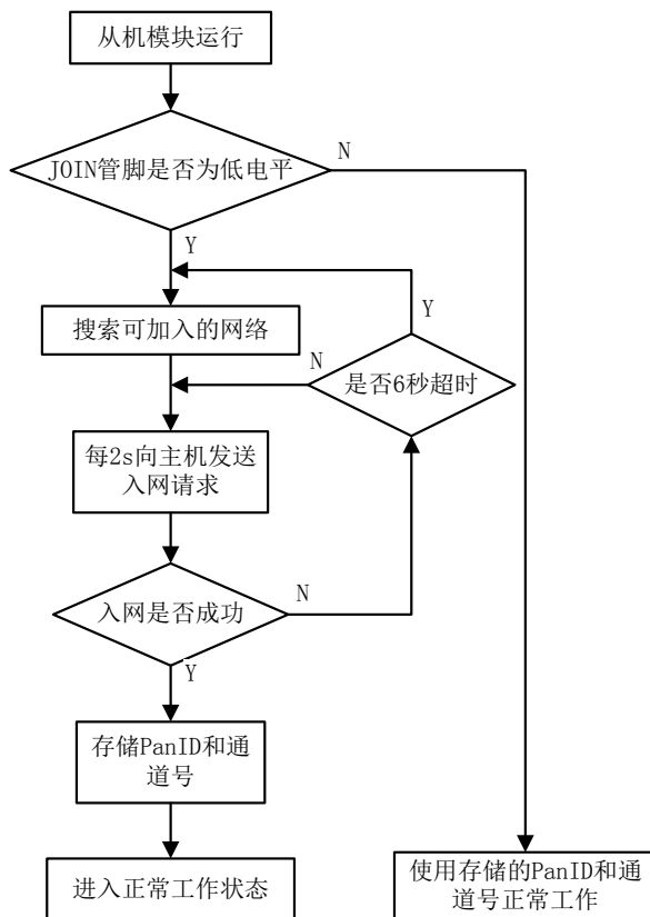
图 14.4 从机模块入网流程
