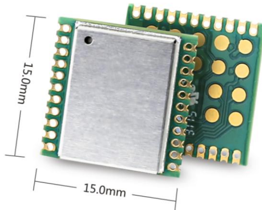
图 1.1 ZM433S-M 正反面
