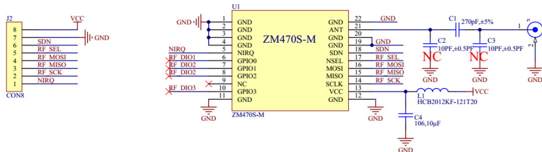
图 7.1 最小系统图
