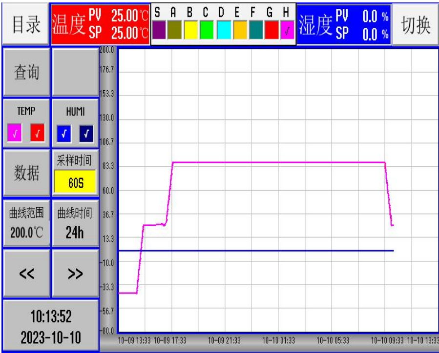
图 6 高温试验曲线
