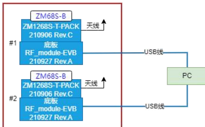
图 2 试验配置框图
