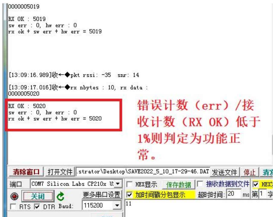
图 4 功能测试
