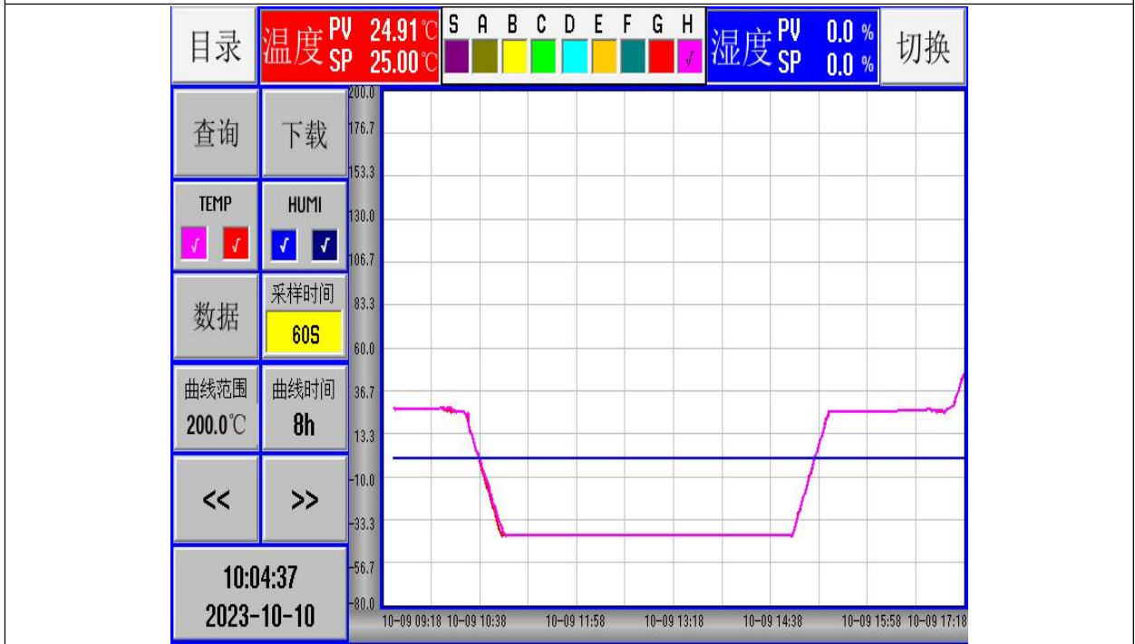
图 5 低温试验曲线
