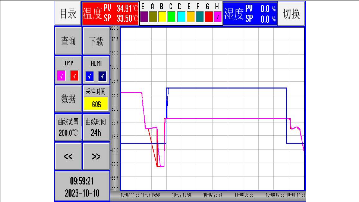
图 8 湿热试验曲线
