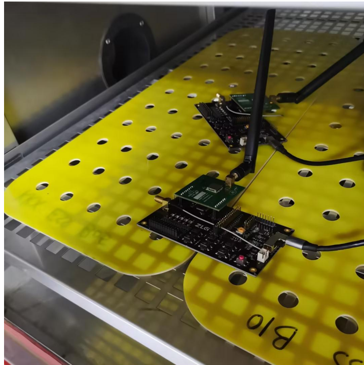
图 3 样机环境试验
