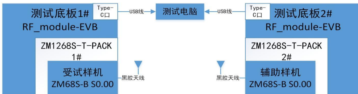
图 1 试验配置示意图
