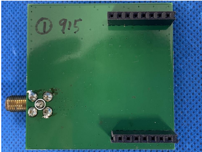
图 7 受试样机 ZM68S-B S0.00 焊接在 ZM1268S-T-PACK 后视图
