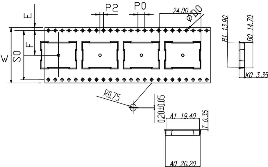
图 7.1 ZM8620 系列模组的载带尺寸
