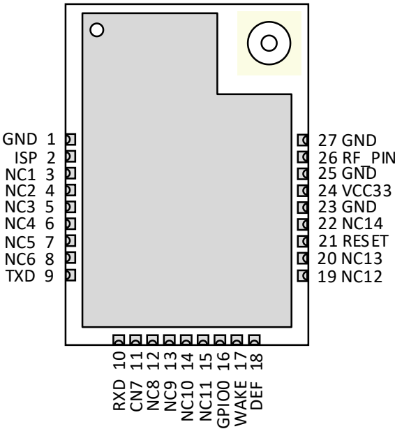
图 3.1 ZM8620 系列模组引脚定义
