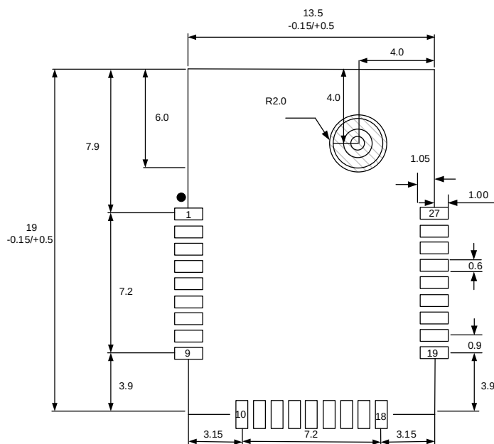
图 5.4 推荐 PCB 封装尺寸
