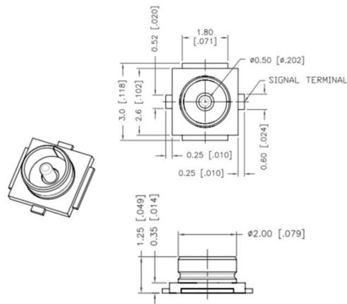
图 5.5 IPEX 连接器参考尺寸图
