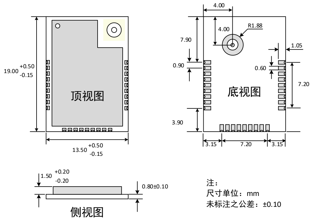
图 2.1 ZM8620 系列模组尺寸图
