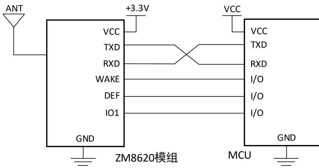
图 5.2 推荐系统应用
