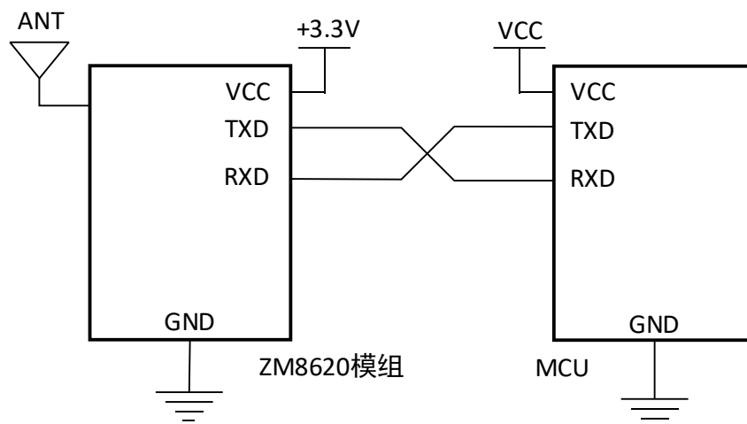
图 5.1 最小系统应用
