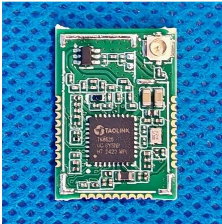
图 5 样机正视图
