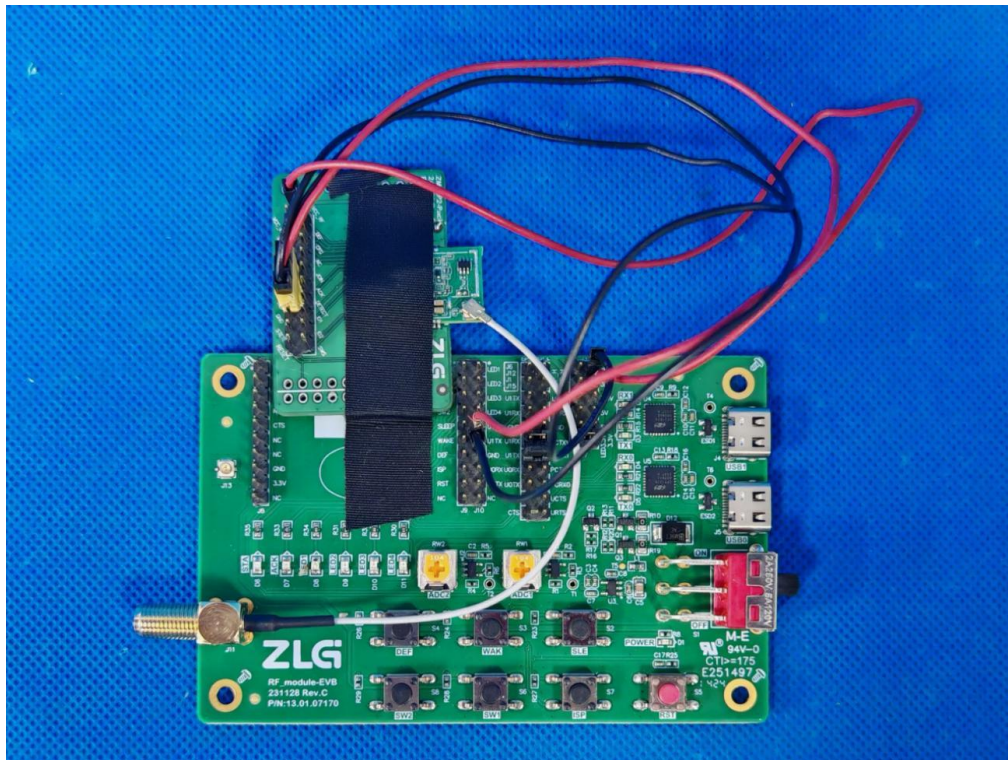
图 7 测试底板正视图
