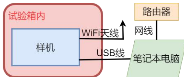
图 2 试验配置框图
