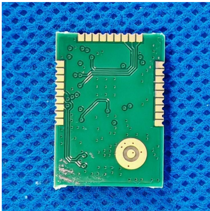
图 6 样机后视图
