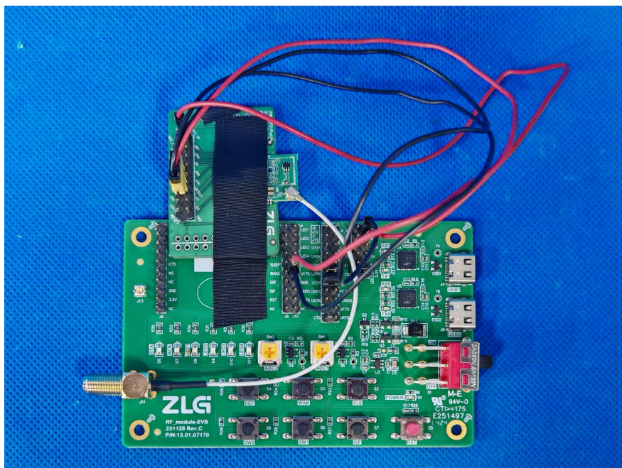
图 5 辅助测试底板正视图
