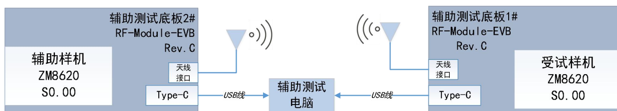
图 1 配置示意图
