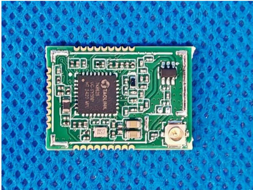
图 4 受试样机 ZM8620 S0.00 正视图
