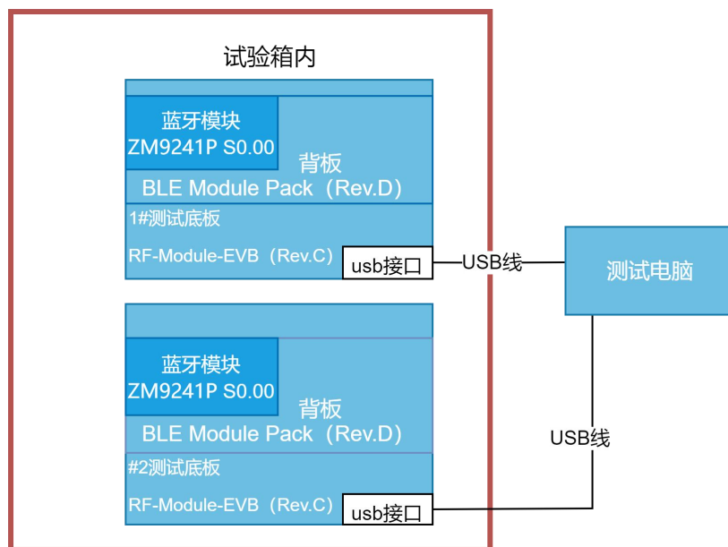
图 2 试验配置框图
