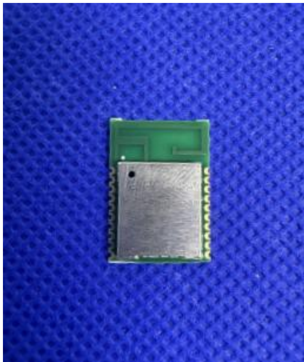
图 5 样机正视图
