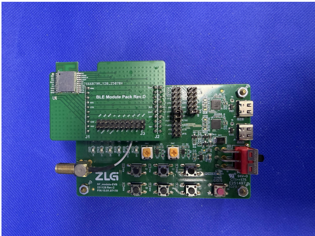
图 7 测试底板正视图
