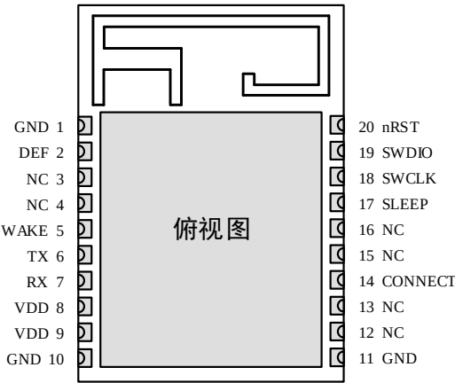
图 3.1 引脚定义
