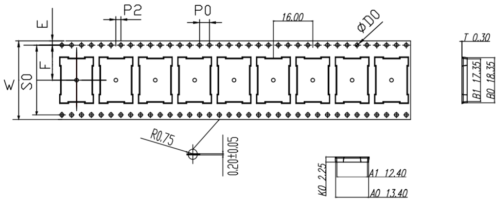
图 7.1 卷带尺寸
