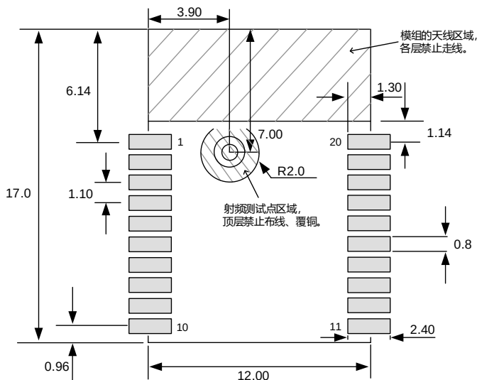
图 5.4 推荐 PCB 封装尺寸
