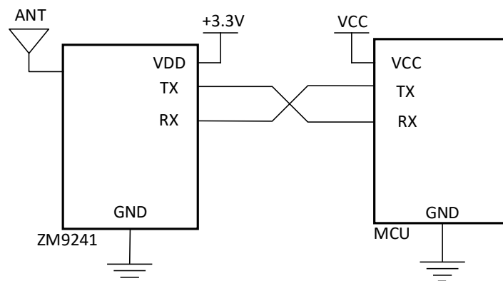
图 5.1 最小系统应用
