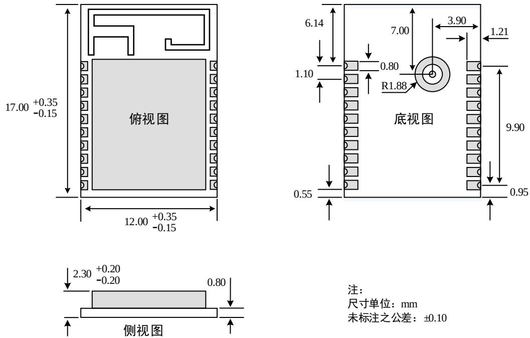
图 2.1 ZM9241 系列模组尺寸图
