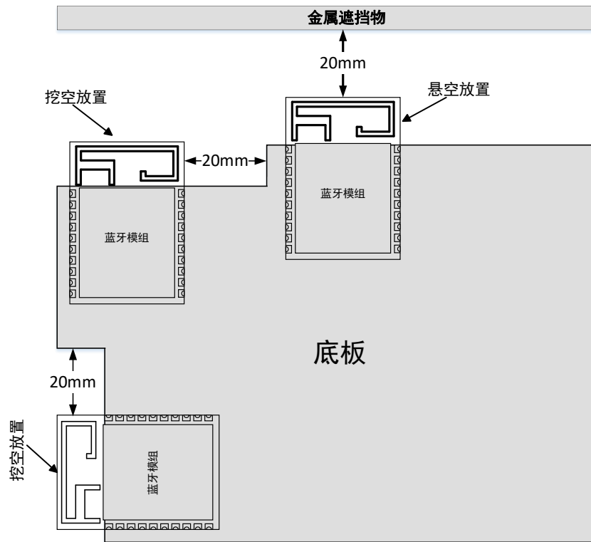
图 5.5 PCB 天线布局指导
