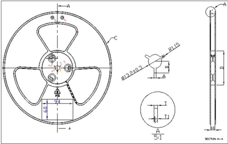
图 7.2 卷盘尺寸
