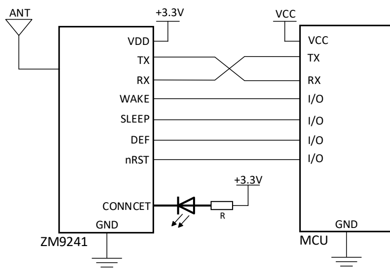
图 5.2 推荐系统应用
