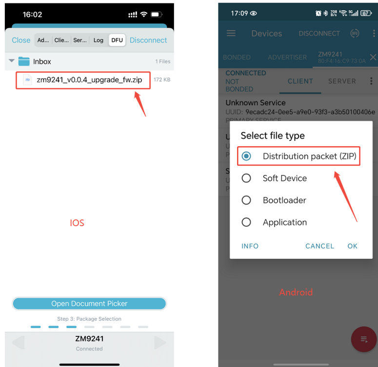
图 5.3 选择固件
