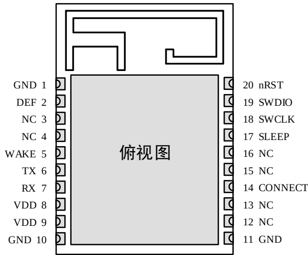
图 2.1 引脚定义
