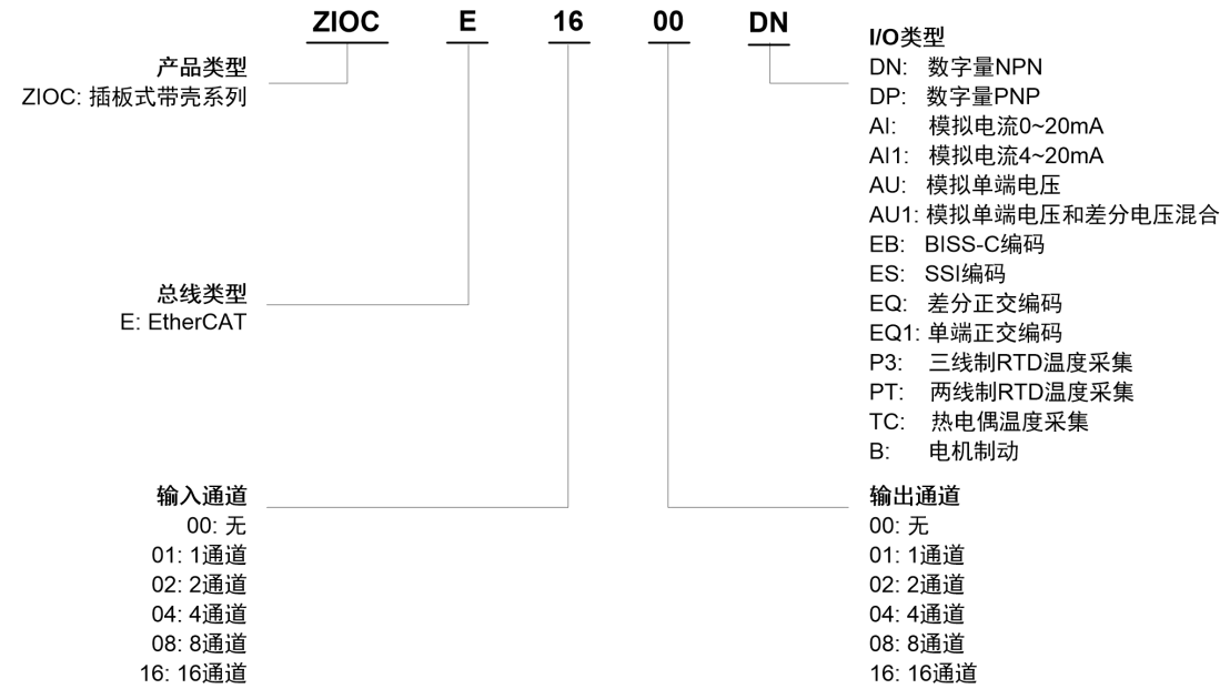
图 2.1 插拔式 I/O 模组选型
