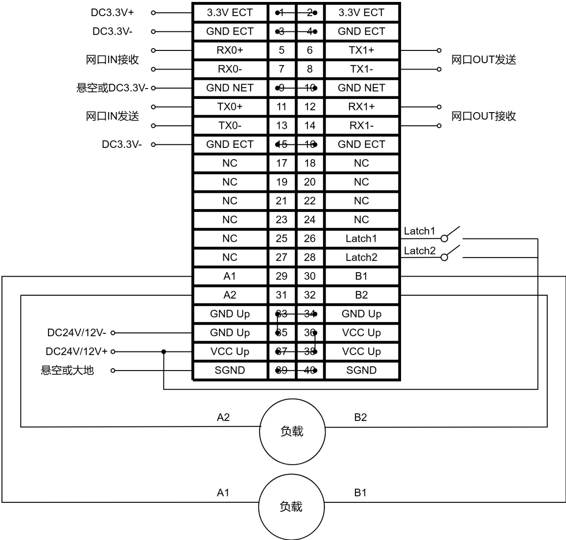
图 4.1 ZIOC-E0002EQ1 典型接线图
