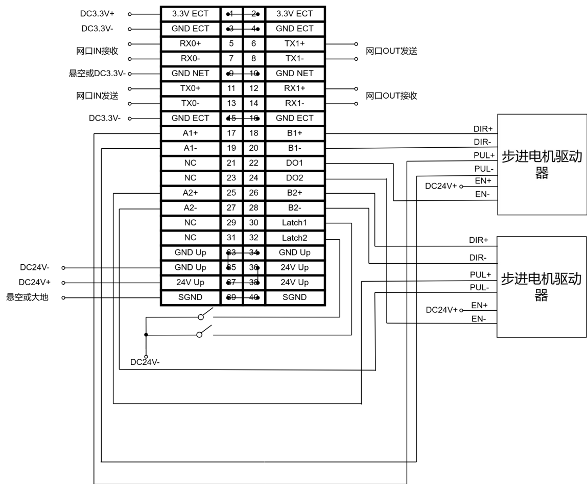
图 4.1 ZIOC-E0002EQ 典型接线图
