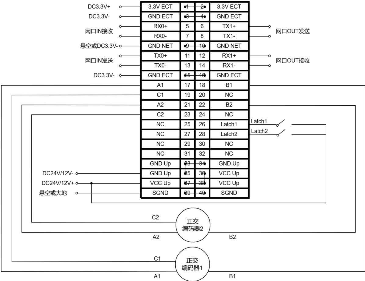
图 4.1 ZIOC-E0200EQ1 典型接线图
