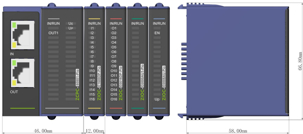
图 3.1 尺寸图
