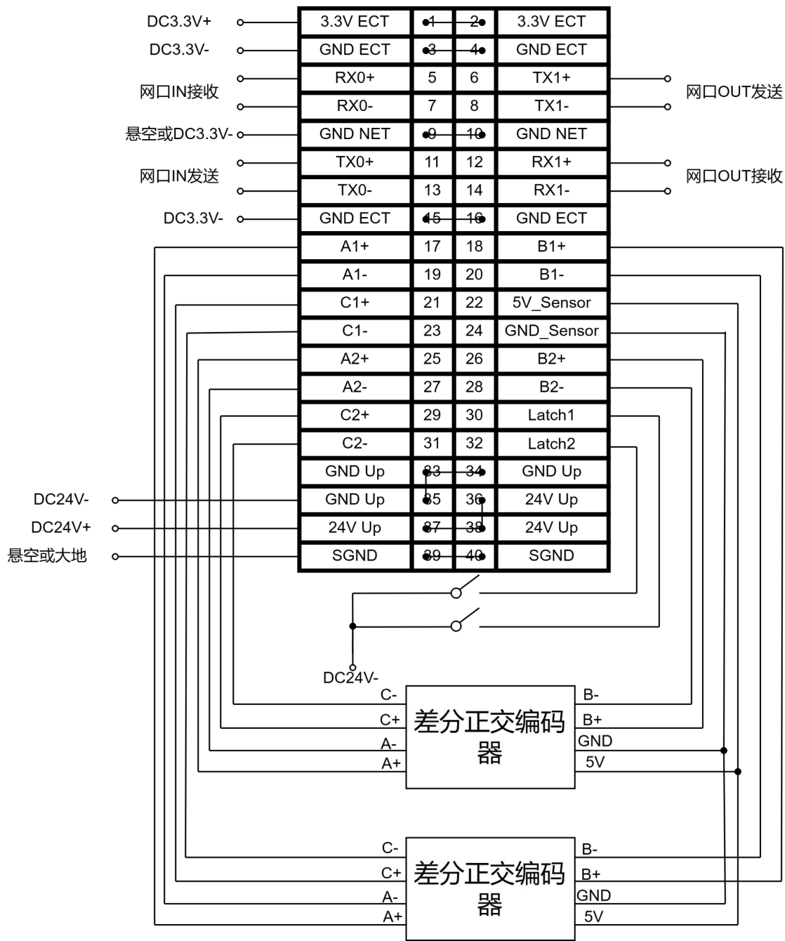
图 4.1 ZIOC-E0200EQ 典型接线图
