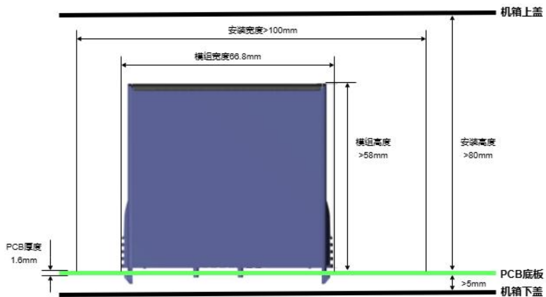
图 3.3 安全距离
