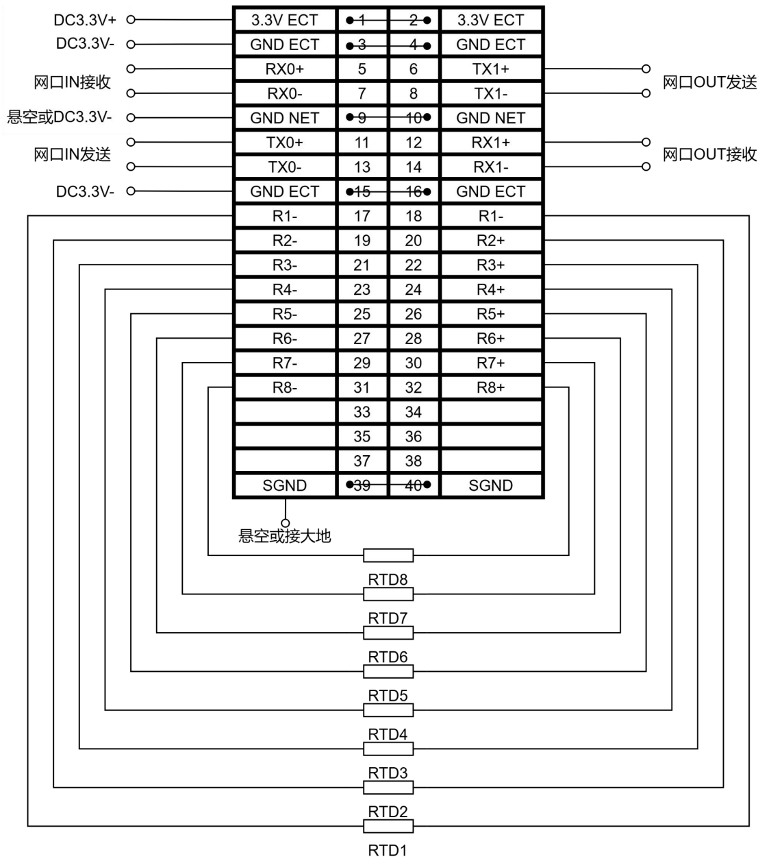
图 4.1 ZIOC-E0800PT 典型接线图
