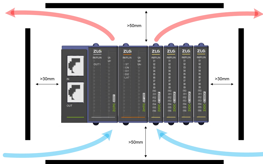
图 3.4 散热空间
