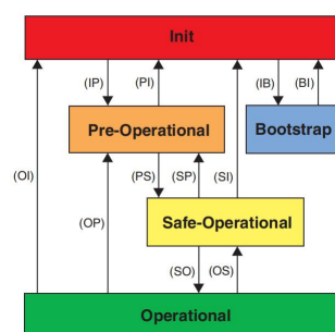
图 5.1 EtherCAT 状态机
