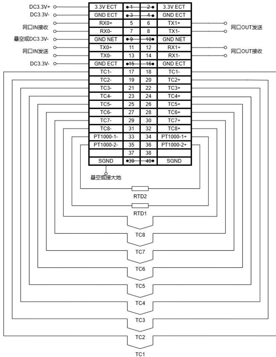
图 4.1 ZIOC-E0800TC 典型接线图
