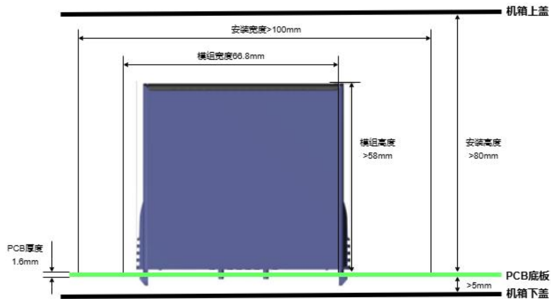
图 3.3 安全距离
