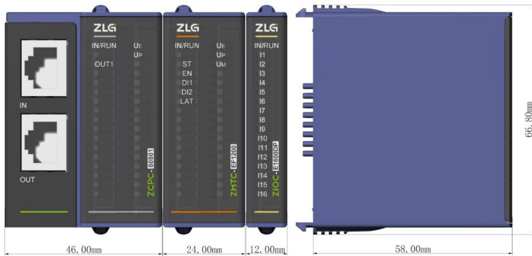
图 3.1 尺寸图
