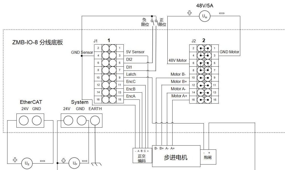
图 4.1 ZMTC-EF1200 步进驱动模组接线
