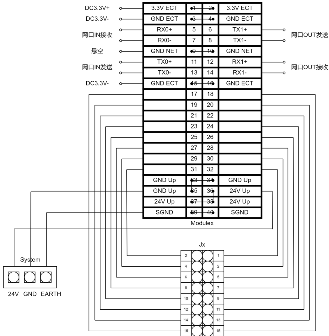
图 3.2 功能模组引线
