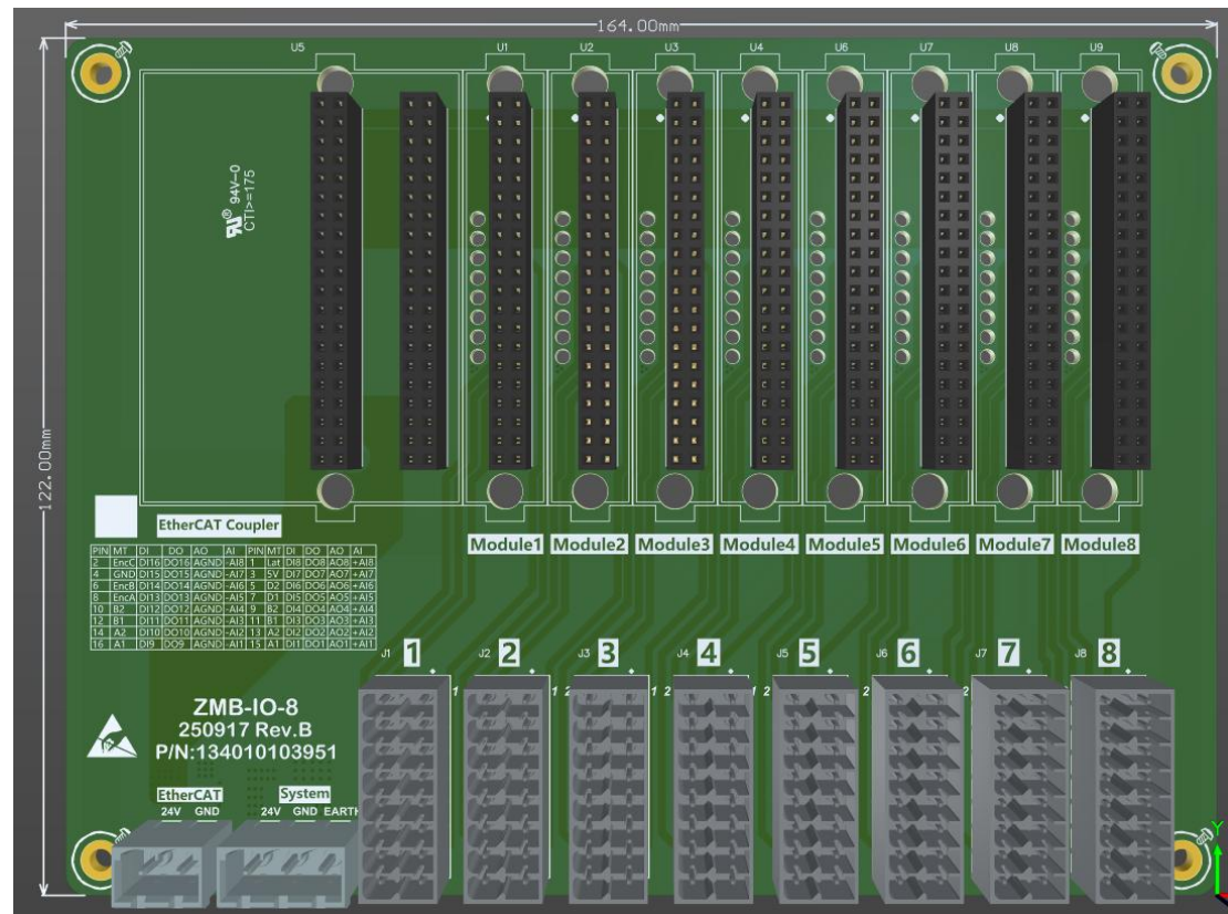
图 3.1 接口位置
