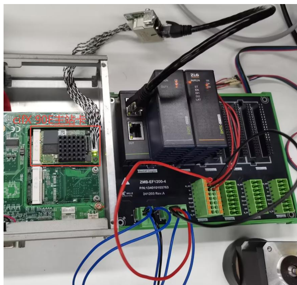
图 4.1 硬件环境
