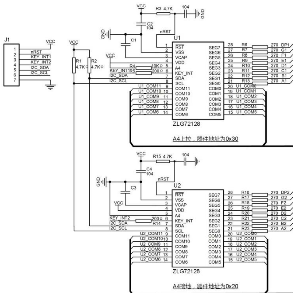
图 1.4 一路 I 2 C 总线上挂接两片 ZLG72128
