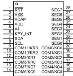
图 1.1 ZLG72128 管脚排列图
