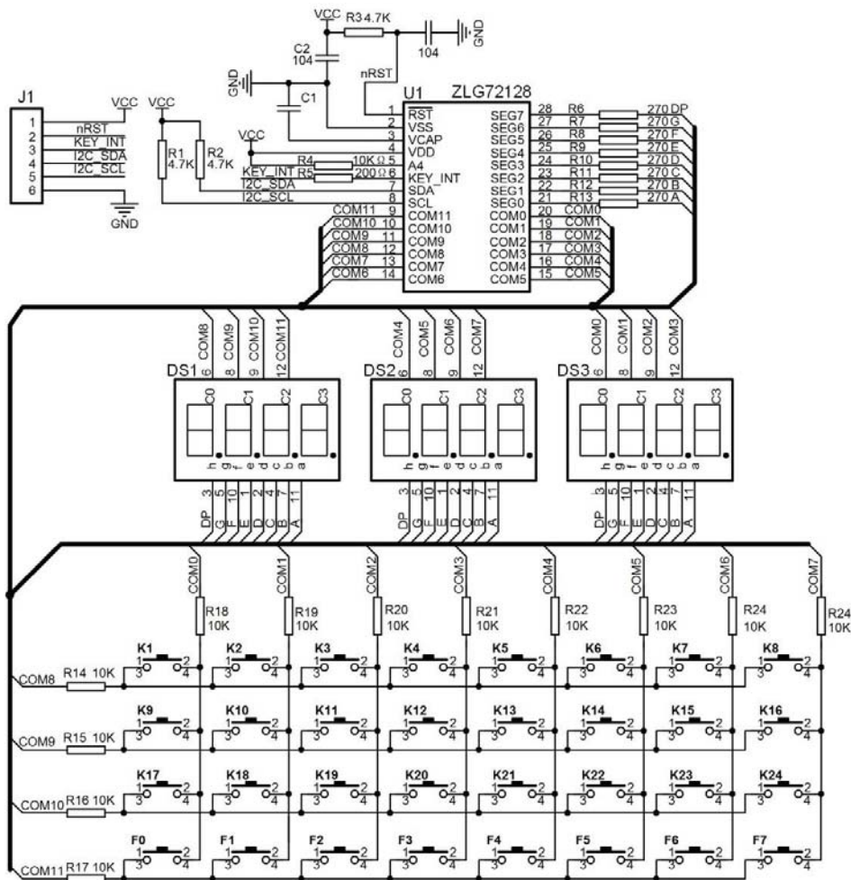
图 1.3 ZLG72128 典型应用电路
